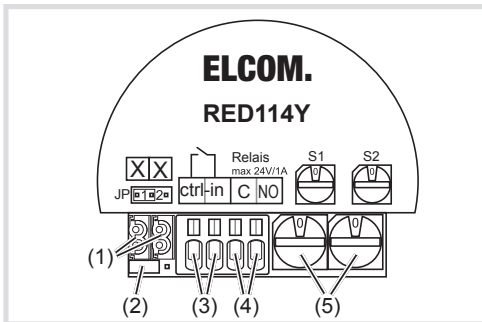
Bild 1: Geräteaufbau
