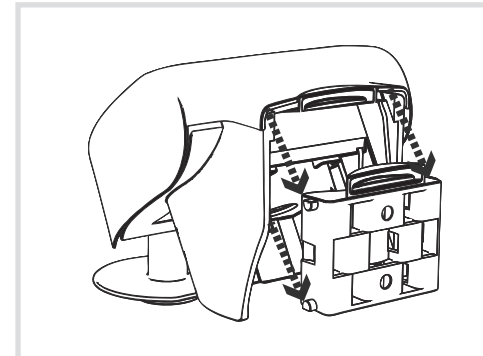
Bild 8: Montage auf Befestigung
