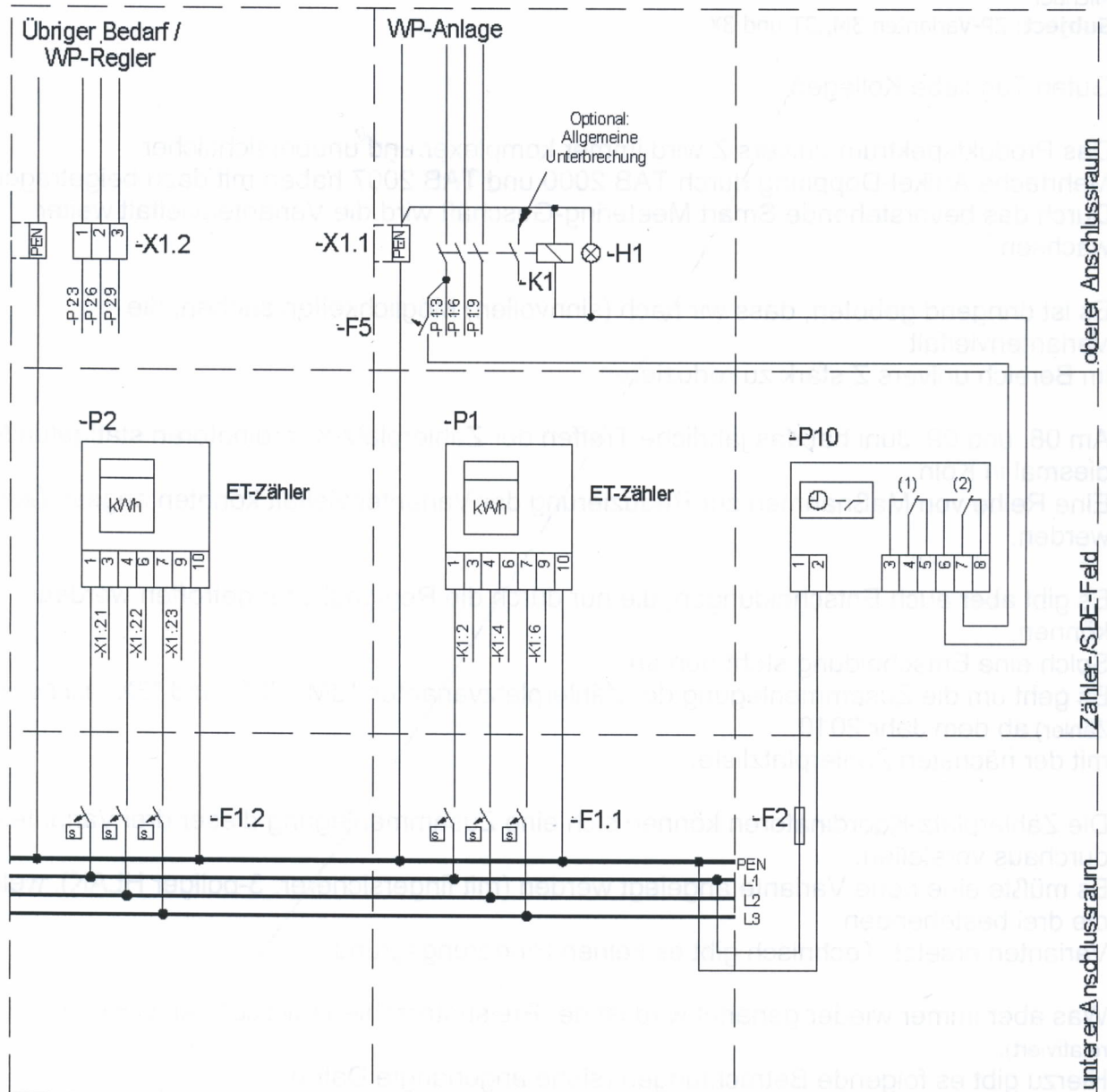
Bild 4.4: Anschaltung für eine Wärmepumpenanlage in variabler Dreipunktbefestigung (2 Kanal-Wochenschaltuhr) (envia NETZ behält sich vor, Tarifsteuergeräte mit abweichender Klemmenbelegung einzusetzen)
