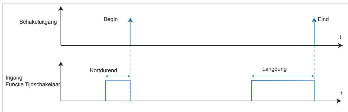
Afbeelding 21: Signaal-tijdschema Tijdschakelaar
