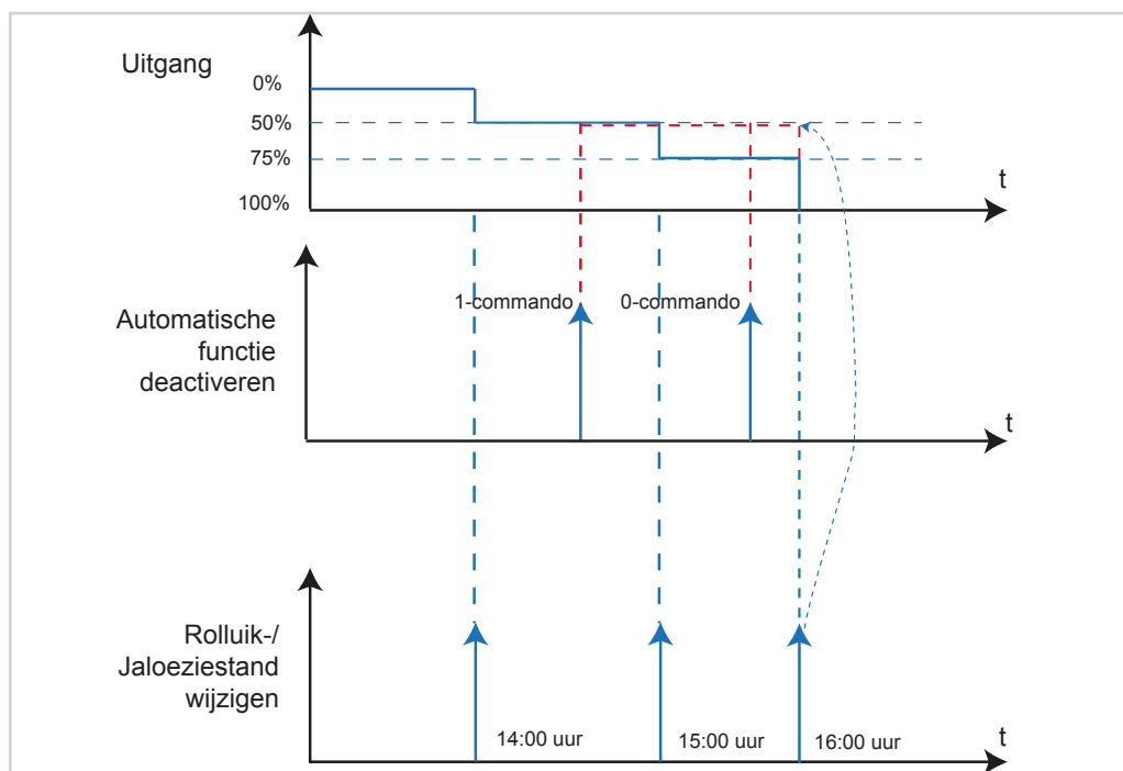
Afbeelding 55: Signaal-tijdschema Automatische functie deactiveren
