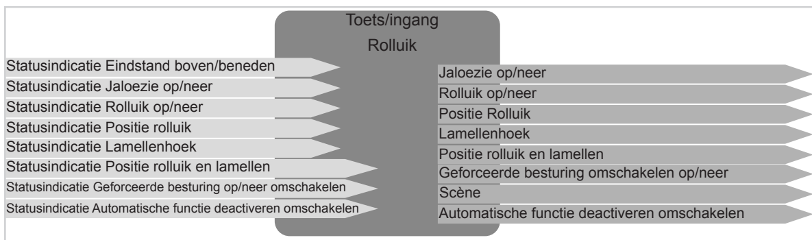
Afbeelding 5: In-/Uitgangssignalen functie rolluik
