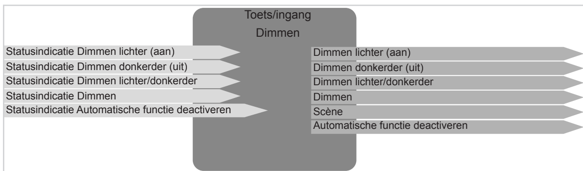
Afbeelding 4: In-/Uitgangssignalen functie Dimmen
