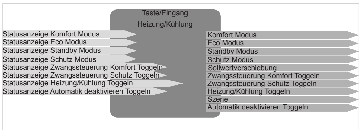
Bild 6: Ein-/Ausgangssignale Funktion Heizung/Kühlung
