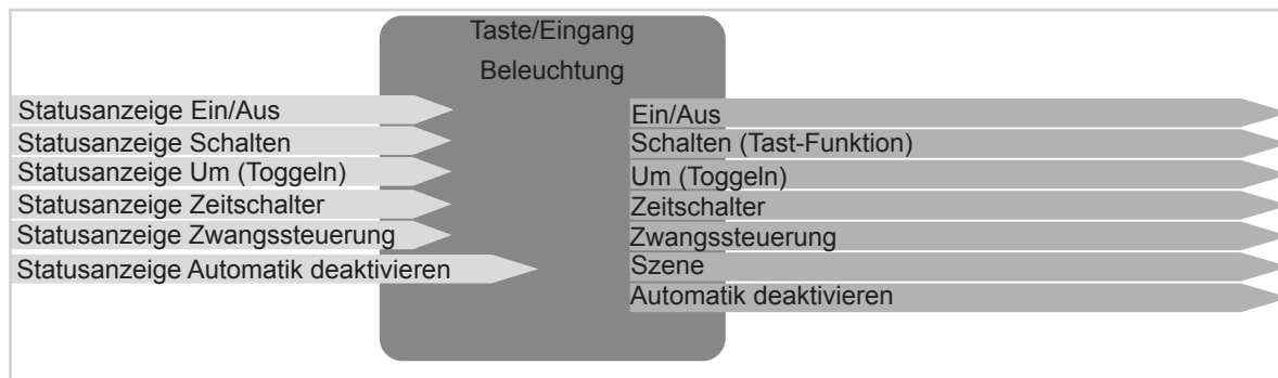
Bild 3: Ein-/Ausgangssignale Funktion Beleuchtung
