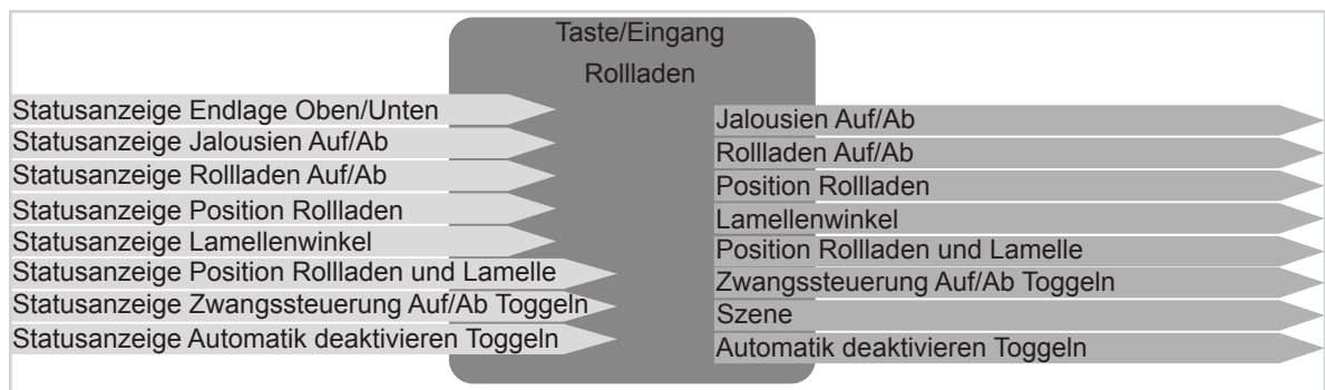
Bild 5: Ein-/Ausgangssignale Funktion Rollläden
