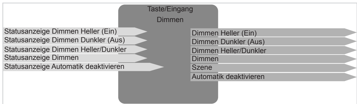
Bild 4: Ein-/Ausgangssignale Funktion Dimmen
