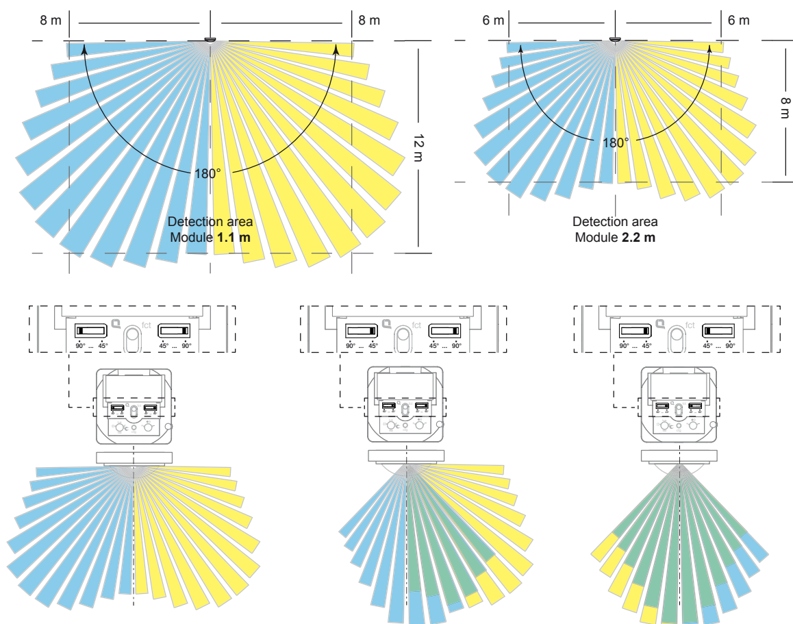
Afbeelding 7: Detectiebereiken
