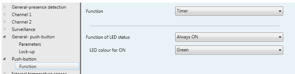
Afbeelding 20: Functie "tijdschakelaar"
