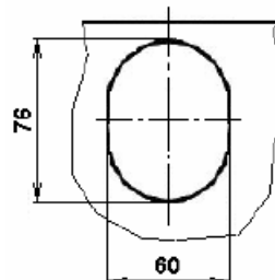
Kabelabgangs- Öffnung (oben)
