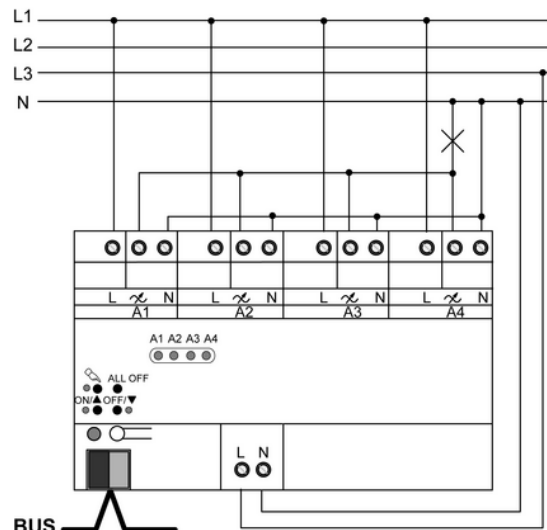
Afbeelding 5: Parallelschakelen van dimuitgangen – aansluitvoorbeeld
