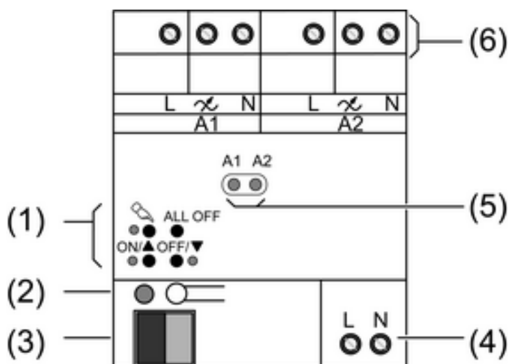
Afbeelding 1: Aanzicht dimactor 2-voudig
