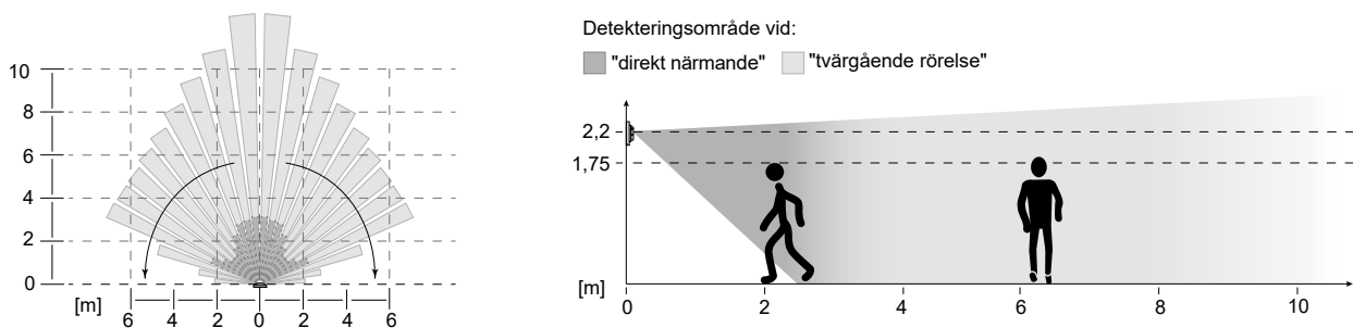
Fig. 7: Rörelsedetektorns detekteringsområde för installationshöjden 2,2 m
