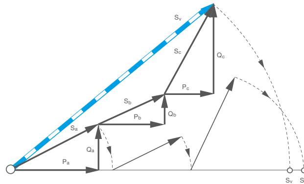
Vektorielle und arithmetische Summierung
