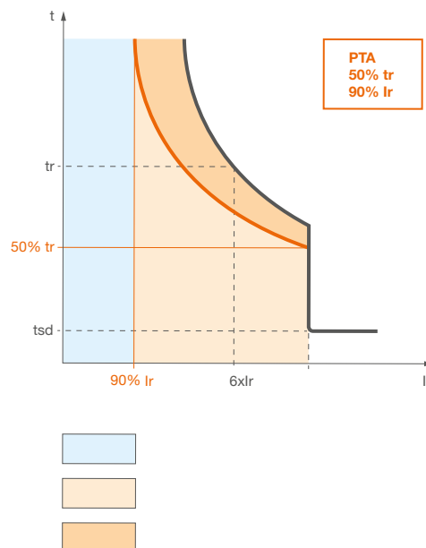
Bereiche des Voralarms bei Überlast
