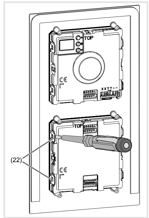
Bild 17: Modul entriegeln
