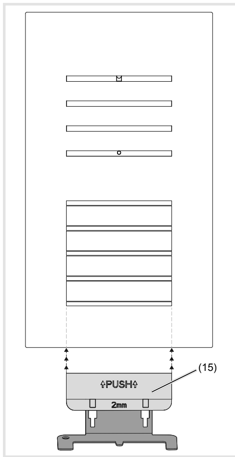
Bild 15: Demontage Türstation
