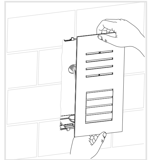
Bild 12: Türstation einsetzen
