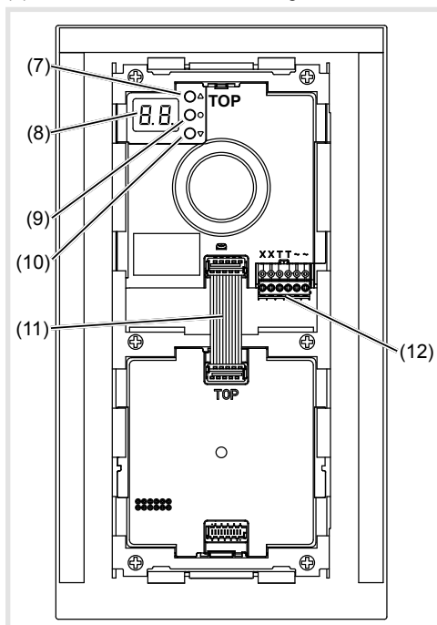
Bild 2: Geräteaufbau Rückseite
