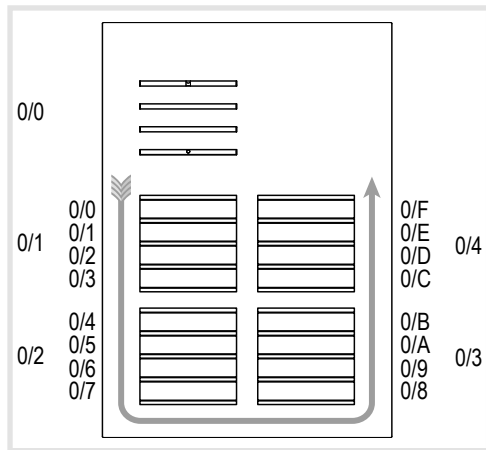
Bild 11: Modul- Adresse und automatische Ruftaster-Adressierung
