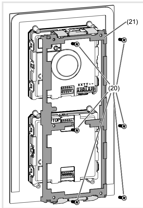
Bild 16: Demontage Modul-Halterung
