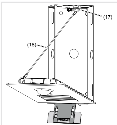
Figura 6: posizione di installazione stazione da porta (17) Fune di sicurezza
