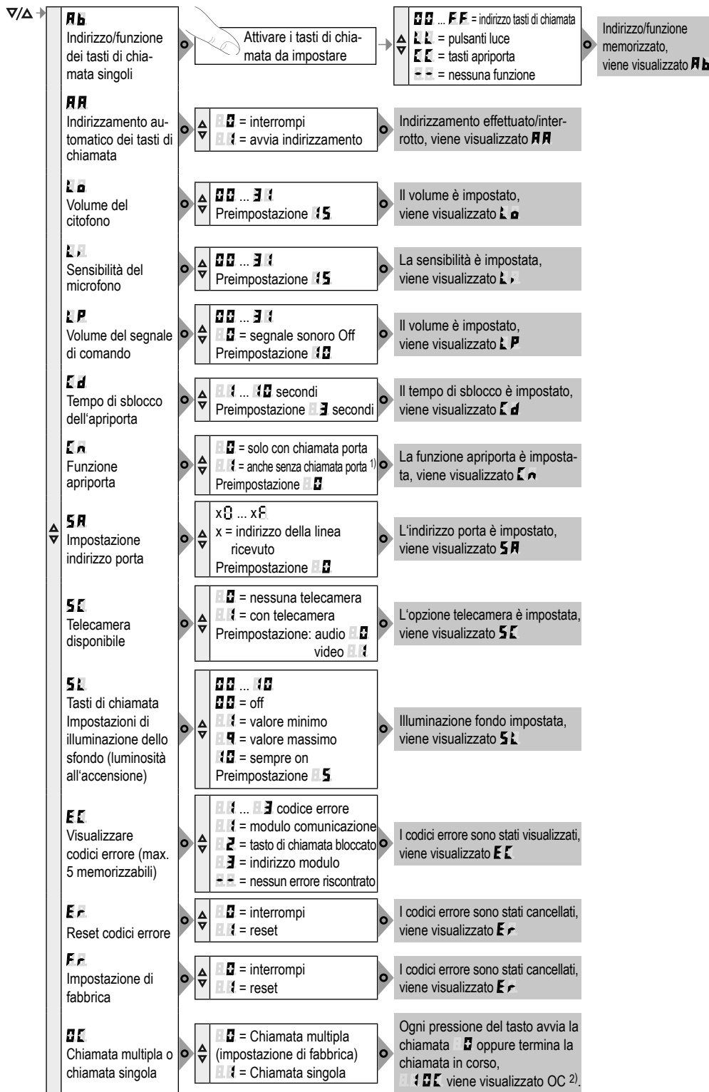
Figura 10: indirizzo modulo e indirizzamento automatico dei tasti di chiamata
