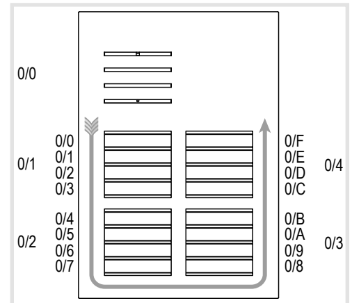
Figura 10: indirizzo modulo e indirizzamento automatico dei tasti di chiamata
