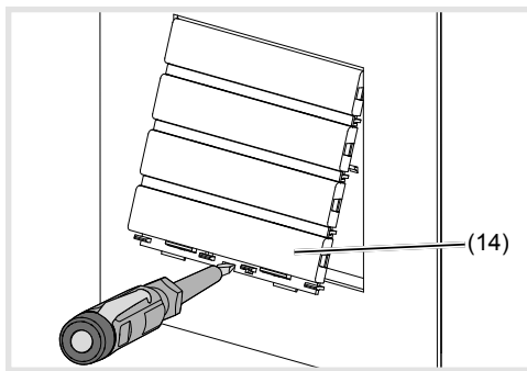
Figura 12: smontaggio mascherina modulo tasti di chiamata
