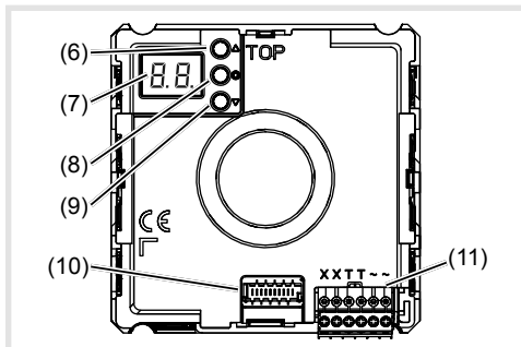
Figura 4: struttura apparecchio moduli audio e mascherina audio, lato posteriore
