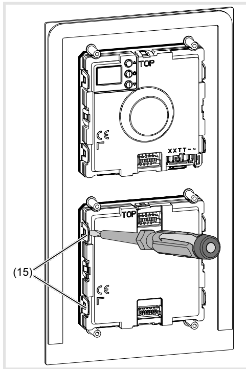
Figura 13: sblocco del modulo
