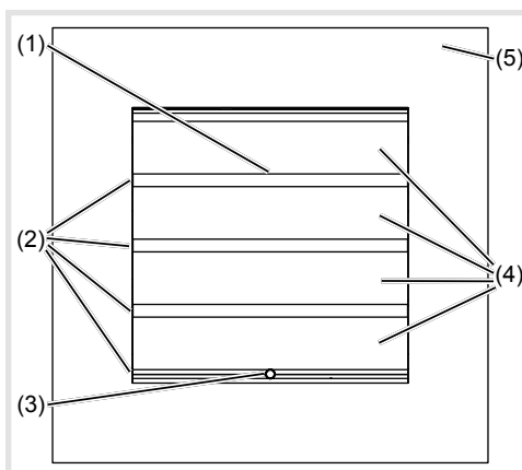
Figura 2: struttura apparecchio modulo audio con portamodulo, lato anteriore
