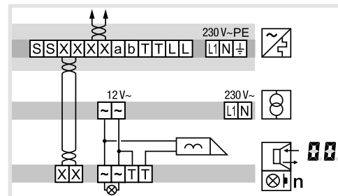
Figura 7: collegamento apriporta della stazione da porta
