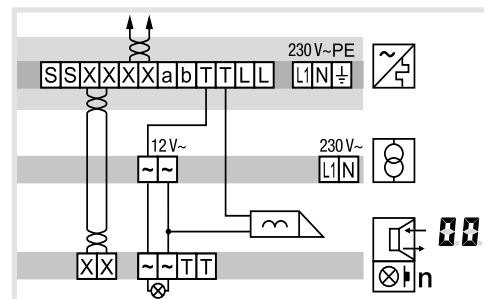
Figura 8: collegamento dell'apparecchio con l'apriporta protetto contro le manomissioni
