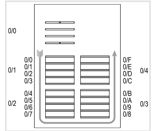
Afb. 10: Module-adres en automatische adressering oproep-toetsen
