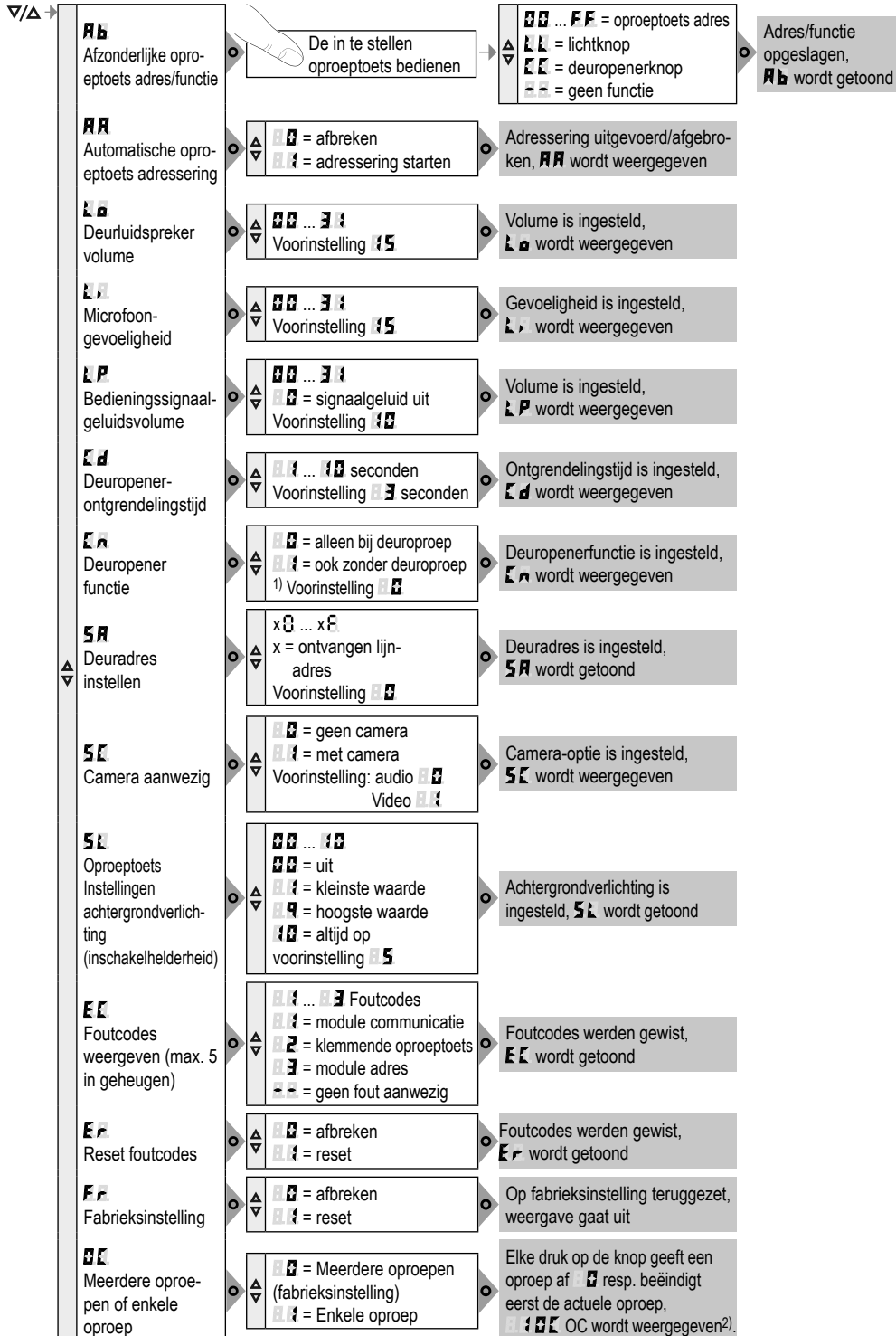
Afb. 10: Module-adres en automatische adressering oproep-toetsen
