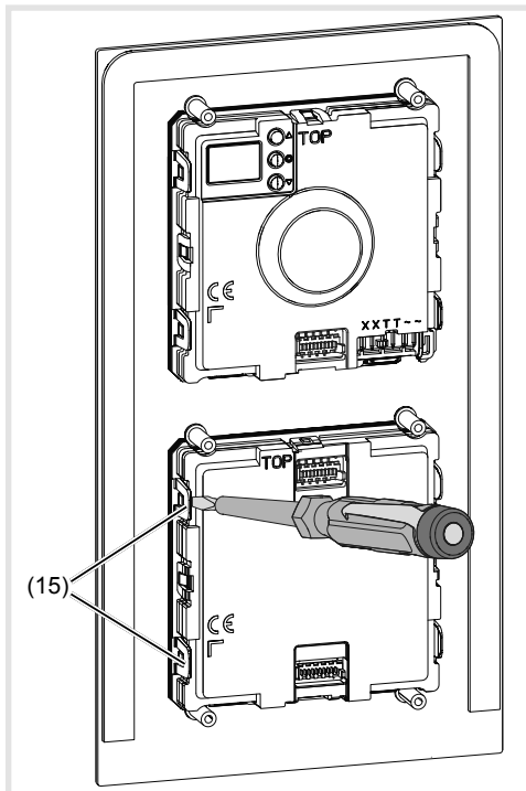
Afb. 13: Module ontgrendelen
