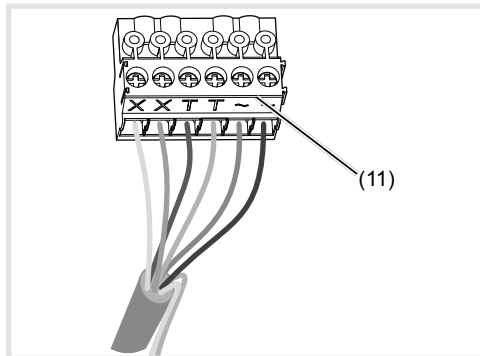
Afb. 6: Bedraad aansluitklemmenblok
