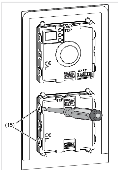
Afb. 13: Module ontgrendelen
