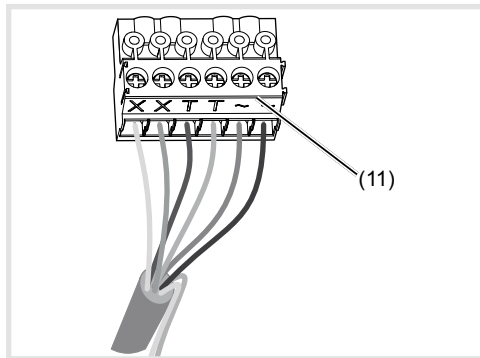
Afb. 6: Bedraad aansluitklemmenblok
