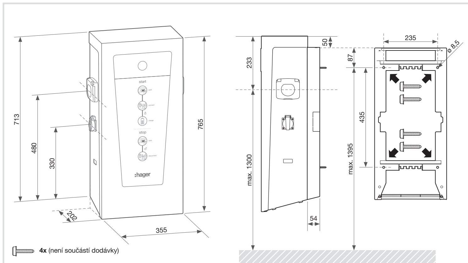
a) Schémata pro vrtání do zdi, s prostorem pro kabeláž na zadní straně, pro model XEV427
