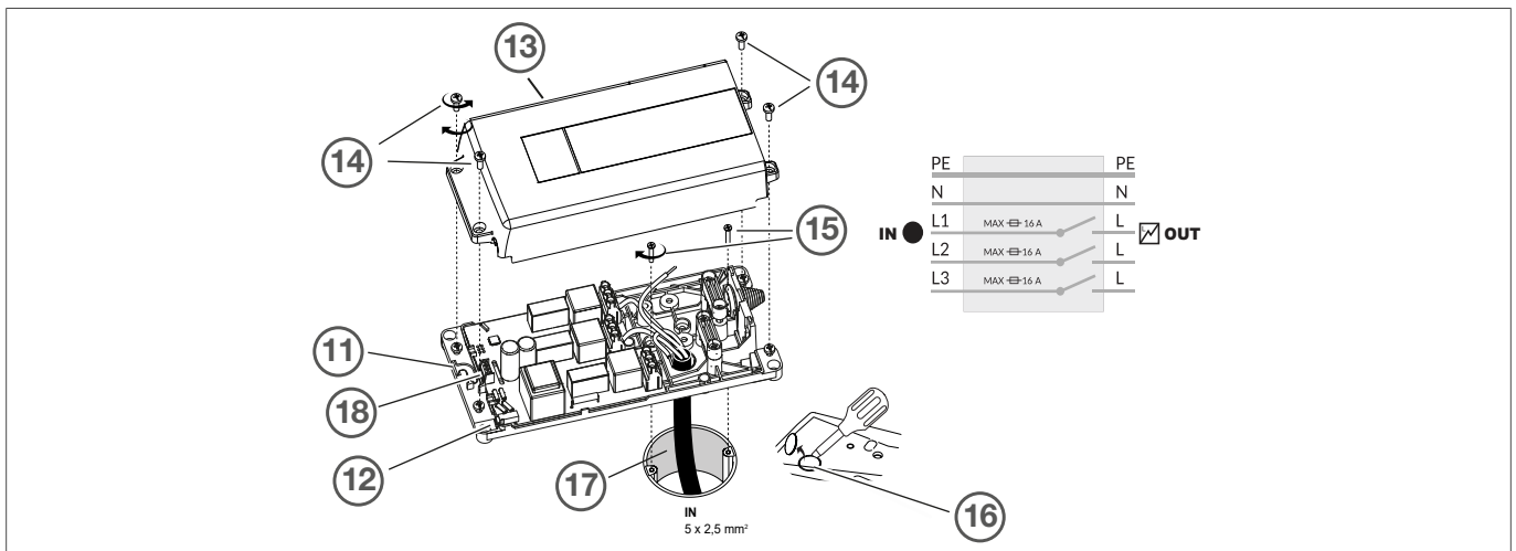
Bild 3: Montage Spannungsunterbrechung
