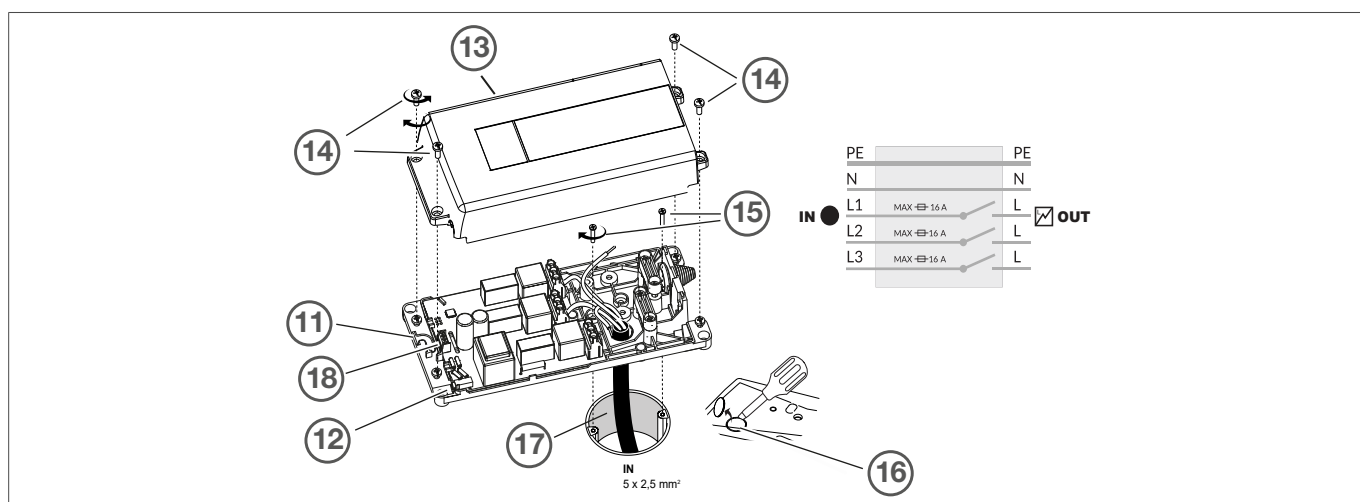
Figure 3: Montage du coupe-tension
