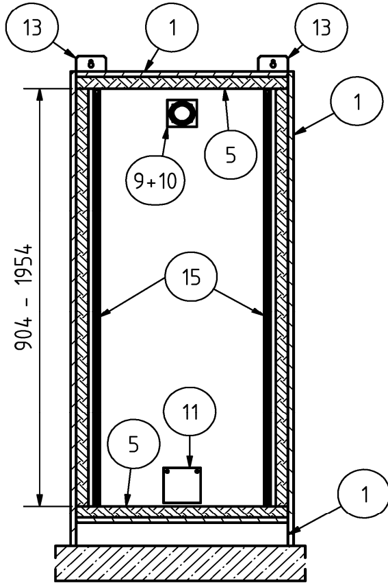
Schnitt C-C
