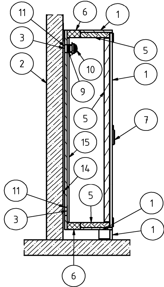
Schnitt B-B
