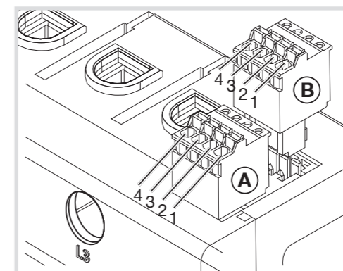
Schéma de raccordement pour connecteur RS485 :
