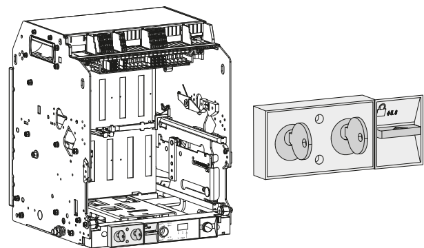
2 Schlösser an der Verriegelungsvorrichtung 1 Lasche zur Positionsverriegelung und Quittierung für Leistungsschalter HW2 und HW4
