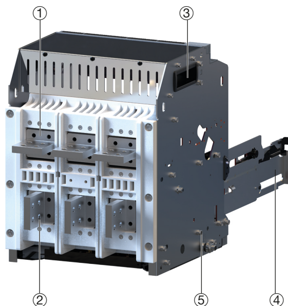
Einschubrahmen für Einschubtechnik-Leistungsschalter HW2 und HW4
