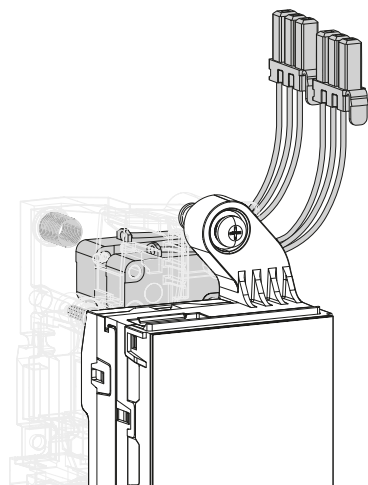
Aufnahme der Fehlermeldek- takte FS
