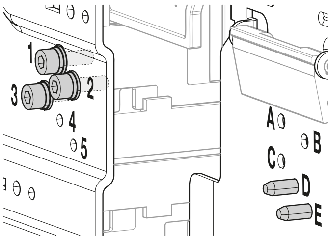
Installationsbeispiel mit den Kombinationen 123 für den Einschubrahmen und DE für den Leistungsschalter HW1.
