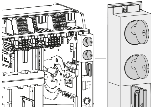
2 Schlösser an der Verriegelungsvorrichtung 1 Lasche zur Positionsverriegelung und Quittierung für Leistungsschalter HW1
