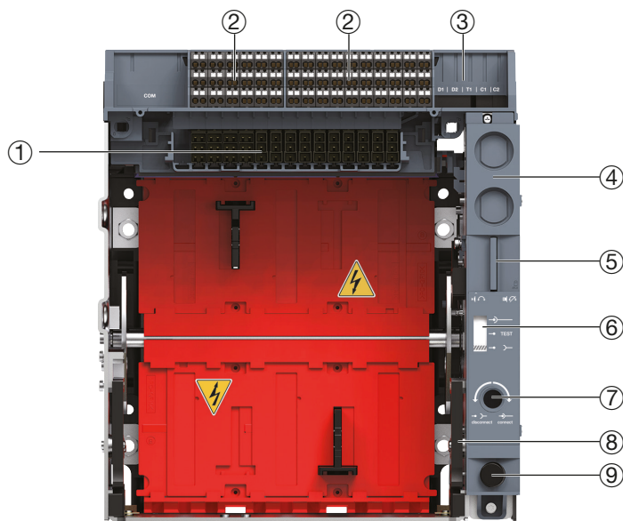
Einschubrahmen für Einschubtechnik-Leistungsschalter HW1
