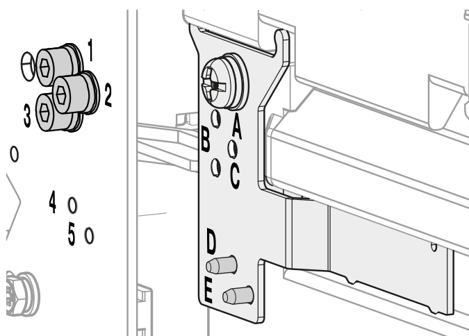
Installationsbeispiel mit den Kombinationen 123 für den Einschubrahmen und DE für die Leistungsschalter HW2, HW4 und HW6.
