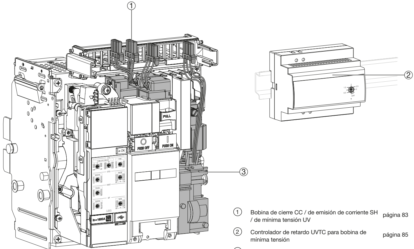
Ejemplo de interruptor automático extraíble
