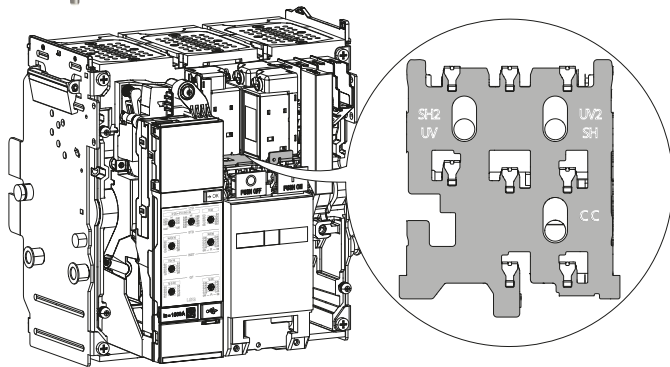
Placa para montaje de bobinas
