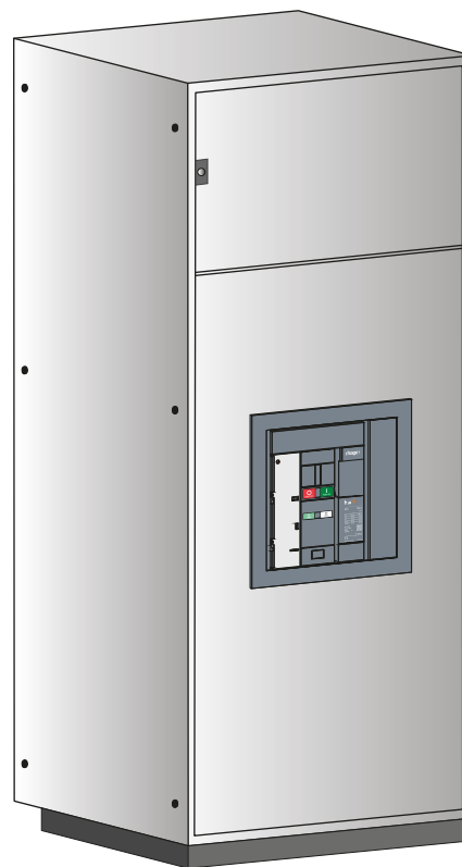
Ejemplos de un marco de la puerta para un interruptor automático fijo HW1
