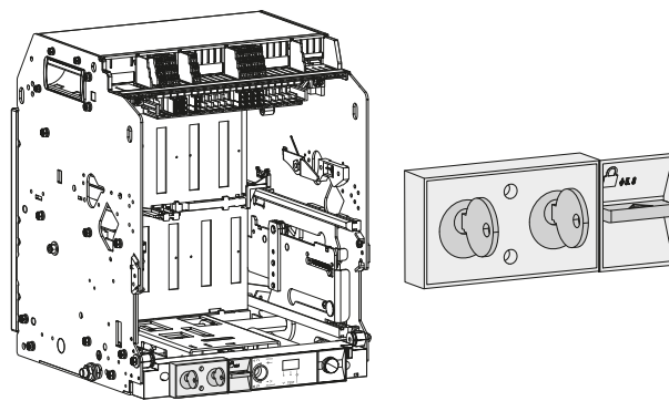
2 cerraduras montadas en el dispositivo de bloqueo 1 cierre por candado y pestaña de reconocimiento de posición para interruptor automático HW2 y HW4.
