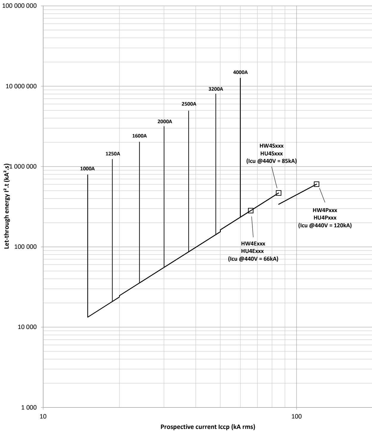
Curva de energía pasante (restricción térmica) 380/440 V AC para HW4
