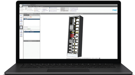
Software Hagercad Software para el diseño y cálculo de costes de los armarios de distribución eléctricos hasta 4000A.
