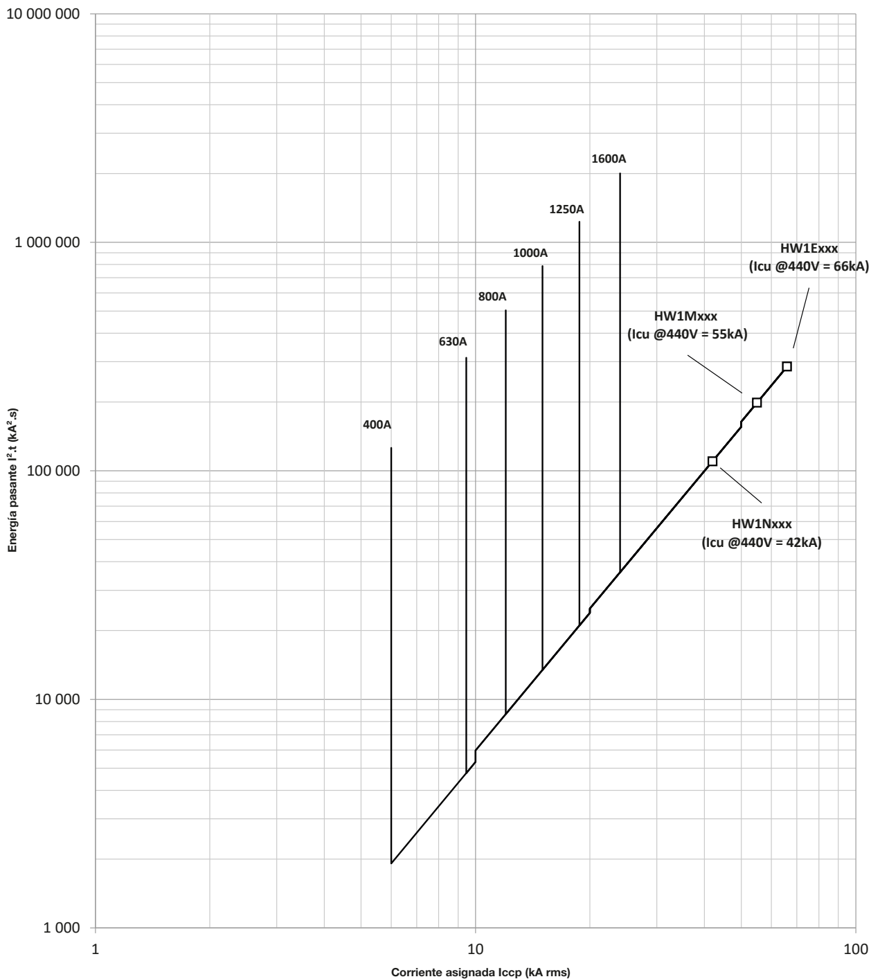
Curva de energía pasante (restricción térmica) 380/440 V AC para HW1
