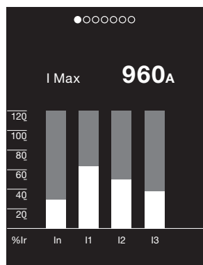
Vue ampèremètre
