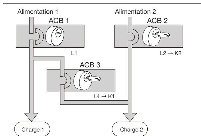
ACB 1 ne peut pas être fermé
