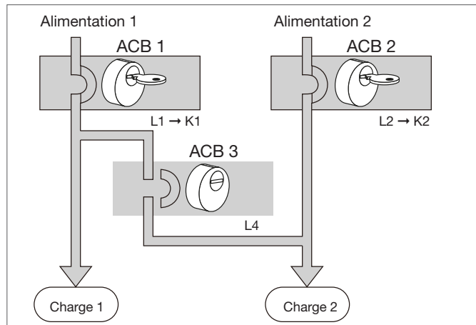
ACB 3 ne peut pas être fermé
