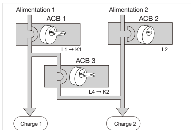
ACB 2 ne peut pas être fermé
