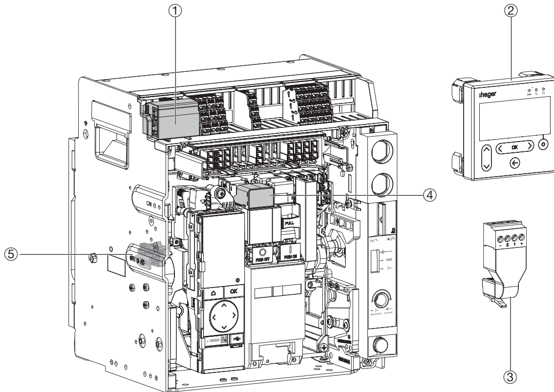
Exemple de disjoncteur débrochable
