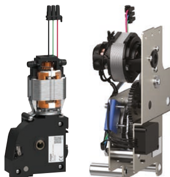
Moteur HW1
