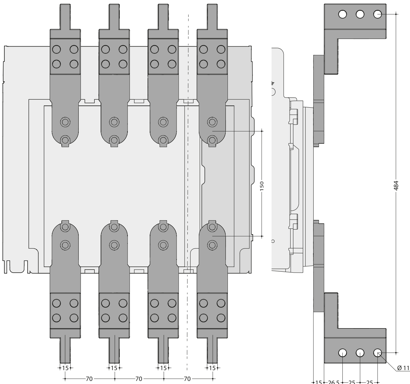
Vista posteriore
