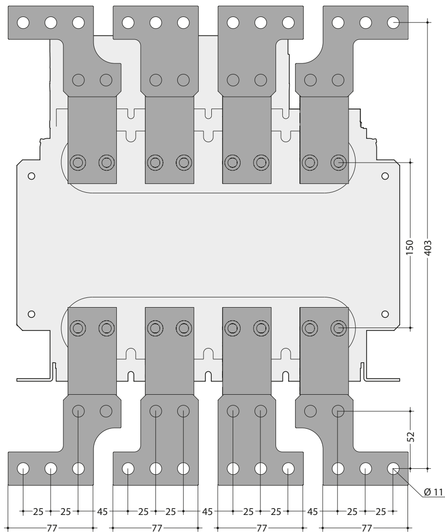
Vista posteriore
