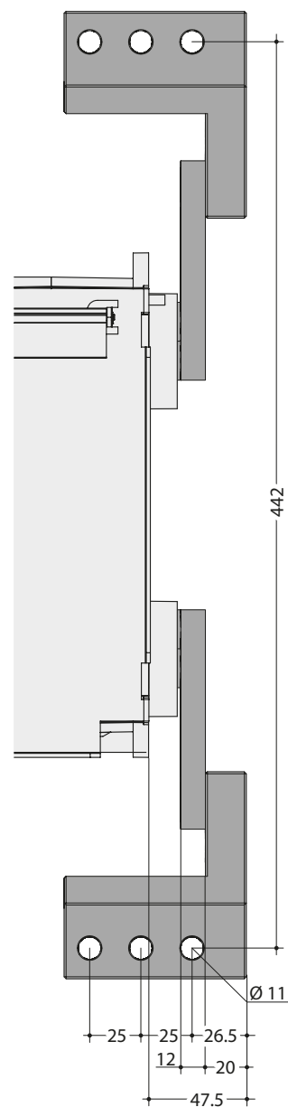
Vista laterale
