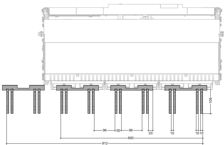
Vista dall'alto
