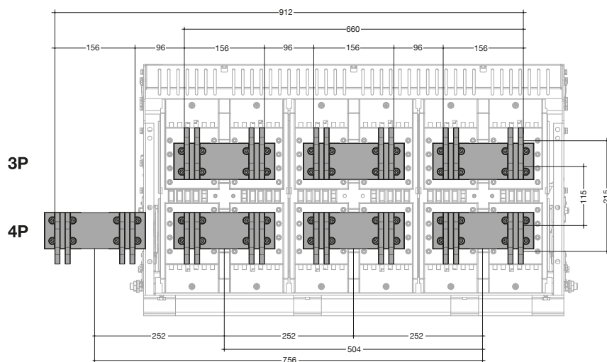
Vista posteriore
