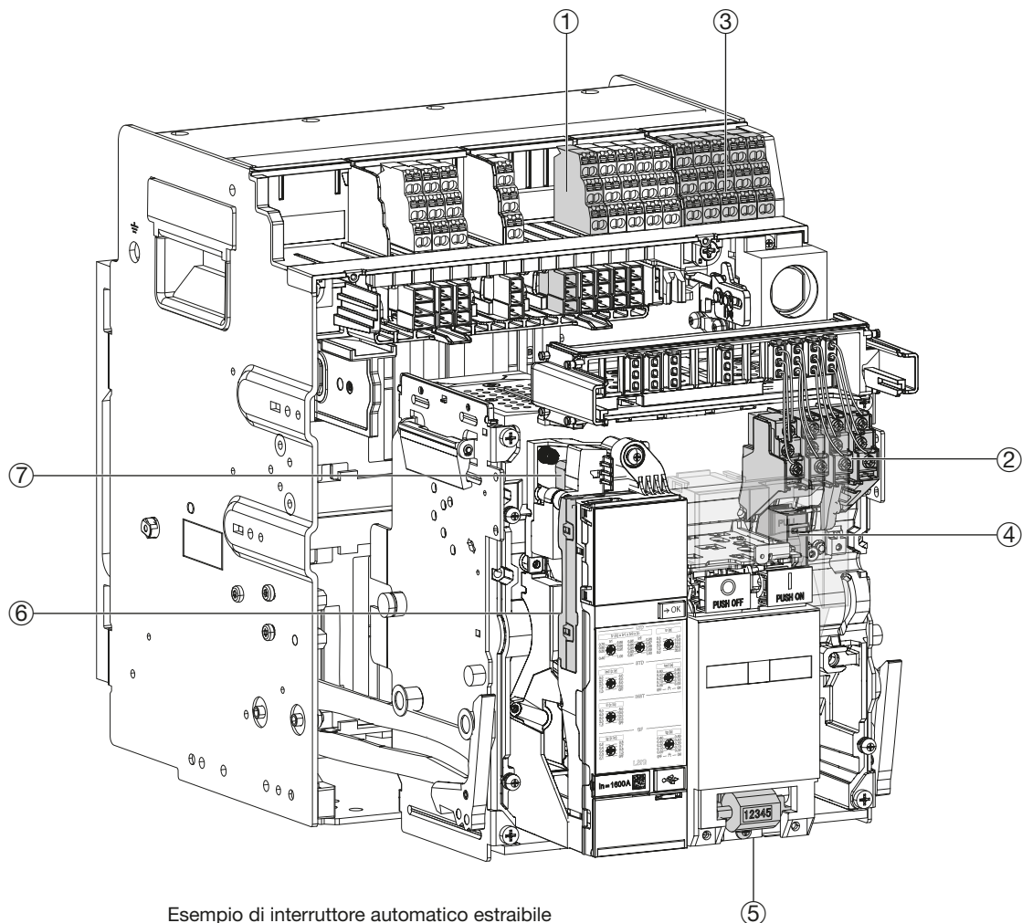
Esempio di interruttore automatico estraibile
