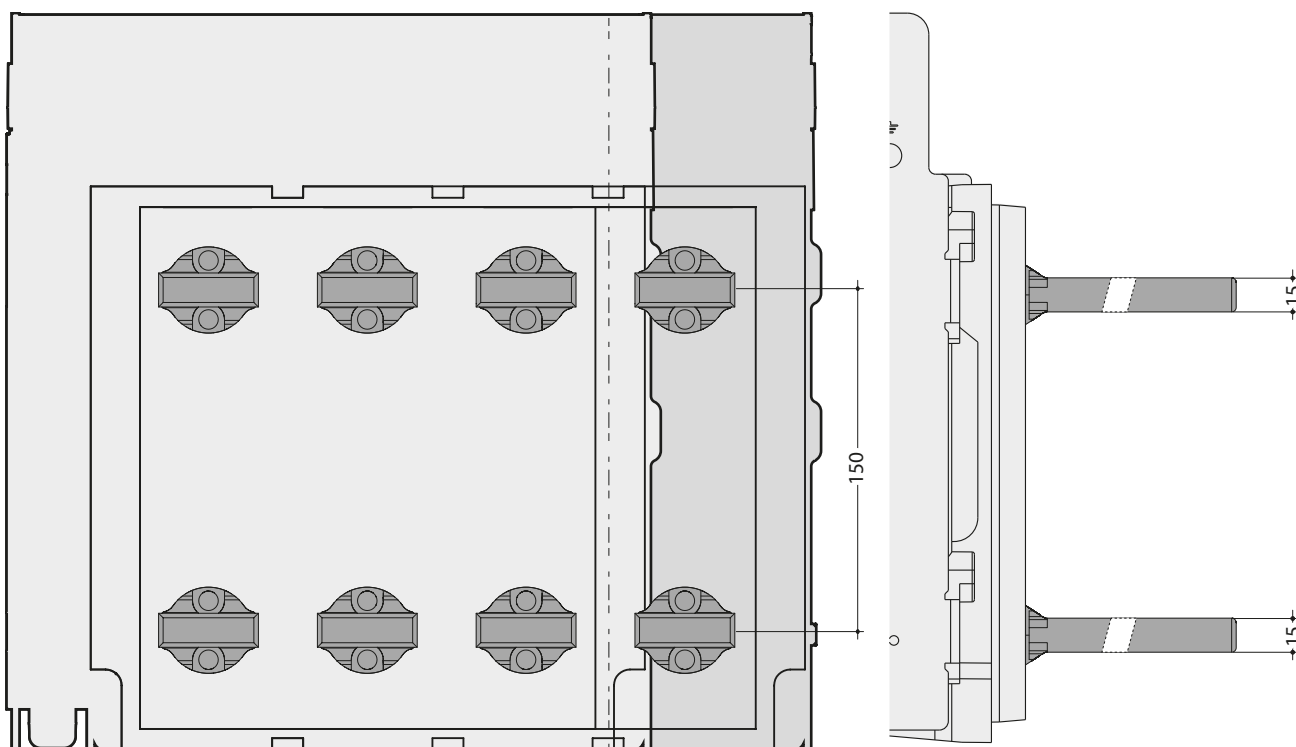
Vista dall'alto
