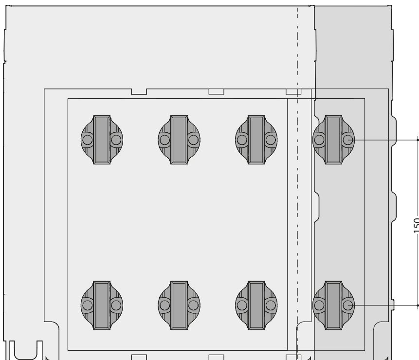
Vista dall'alto
