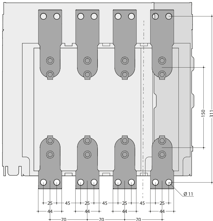
Vista posteriore
