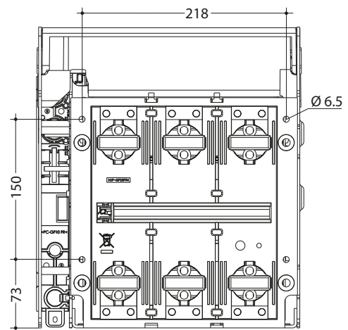
Vista posteriore
