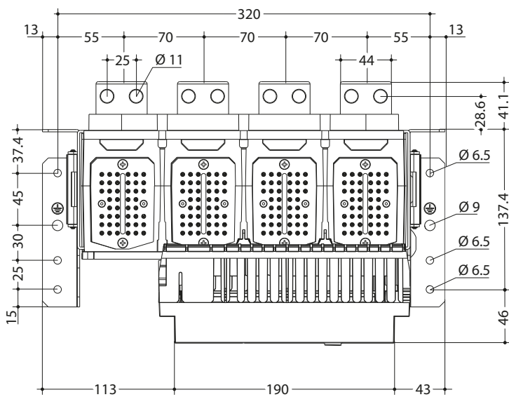
Vista dall'alto
