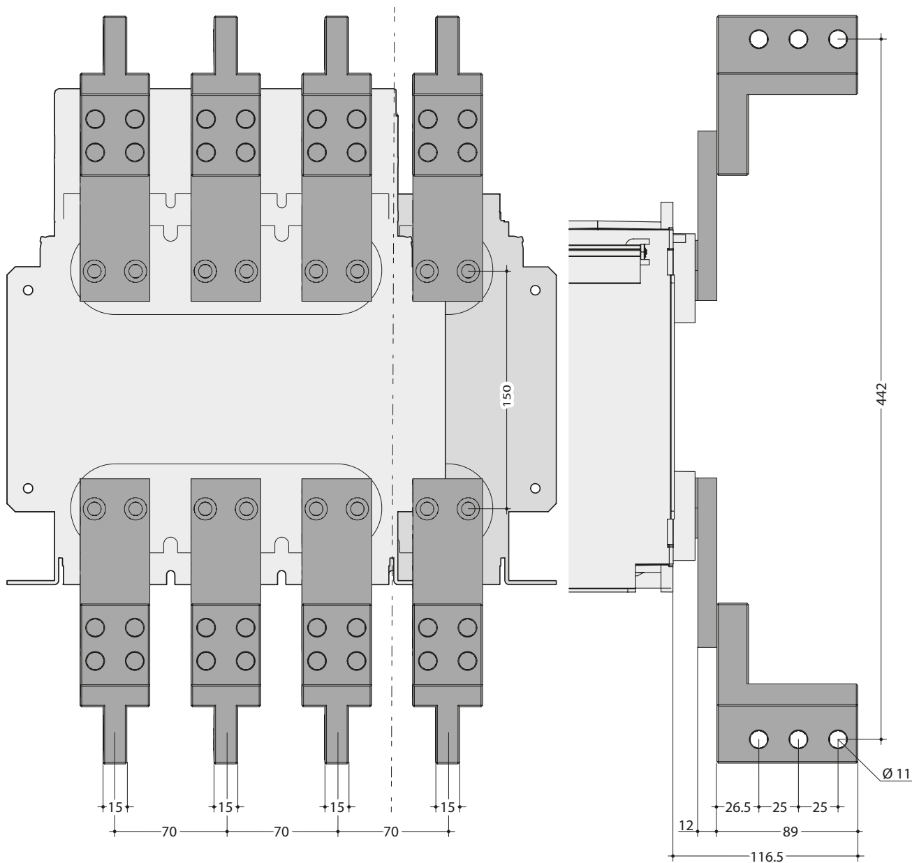
Vista posteriore
