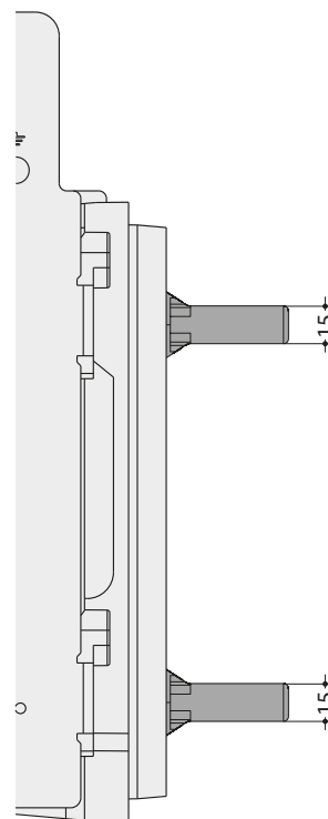
Vista laterale
