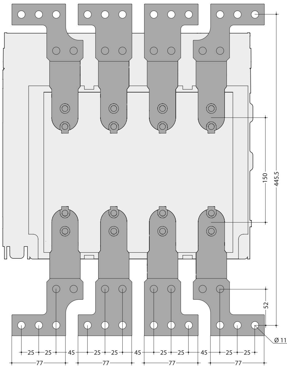
Vista posteriore
