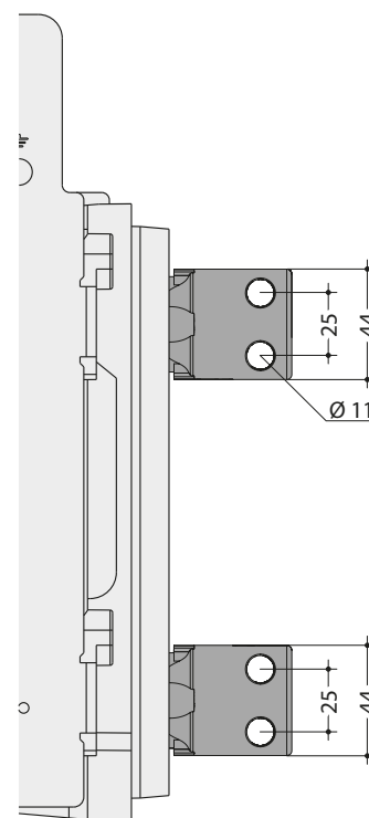
Vista laterale
