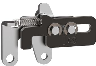
Blocco inserzione porta aperta RI HW1
