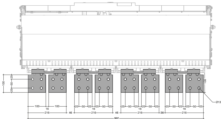
Vista dall'alto
