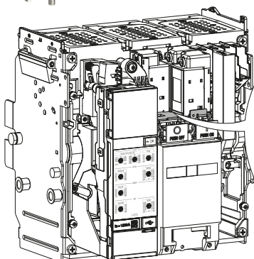
Piastra per alloggiamento delle bobine
