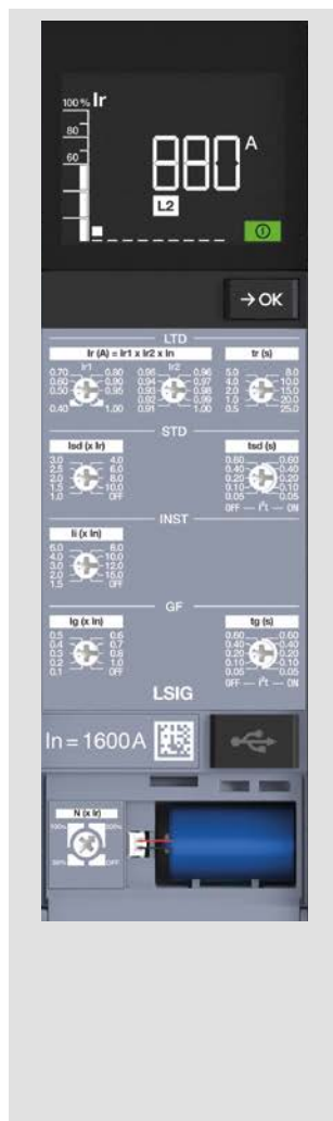
Lectura de corriente en la fase con mayor carga L1, L2 o L3 y como porcentaje del ajuste Ir.
