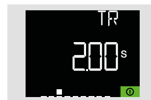
Ajuste del retardo de larga duración.
