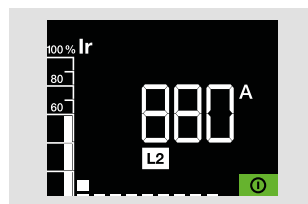
Lectura de corriente en la fase con mayor carga L1, L2 o L3 y como porcentaje del ajuste Ir.
