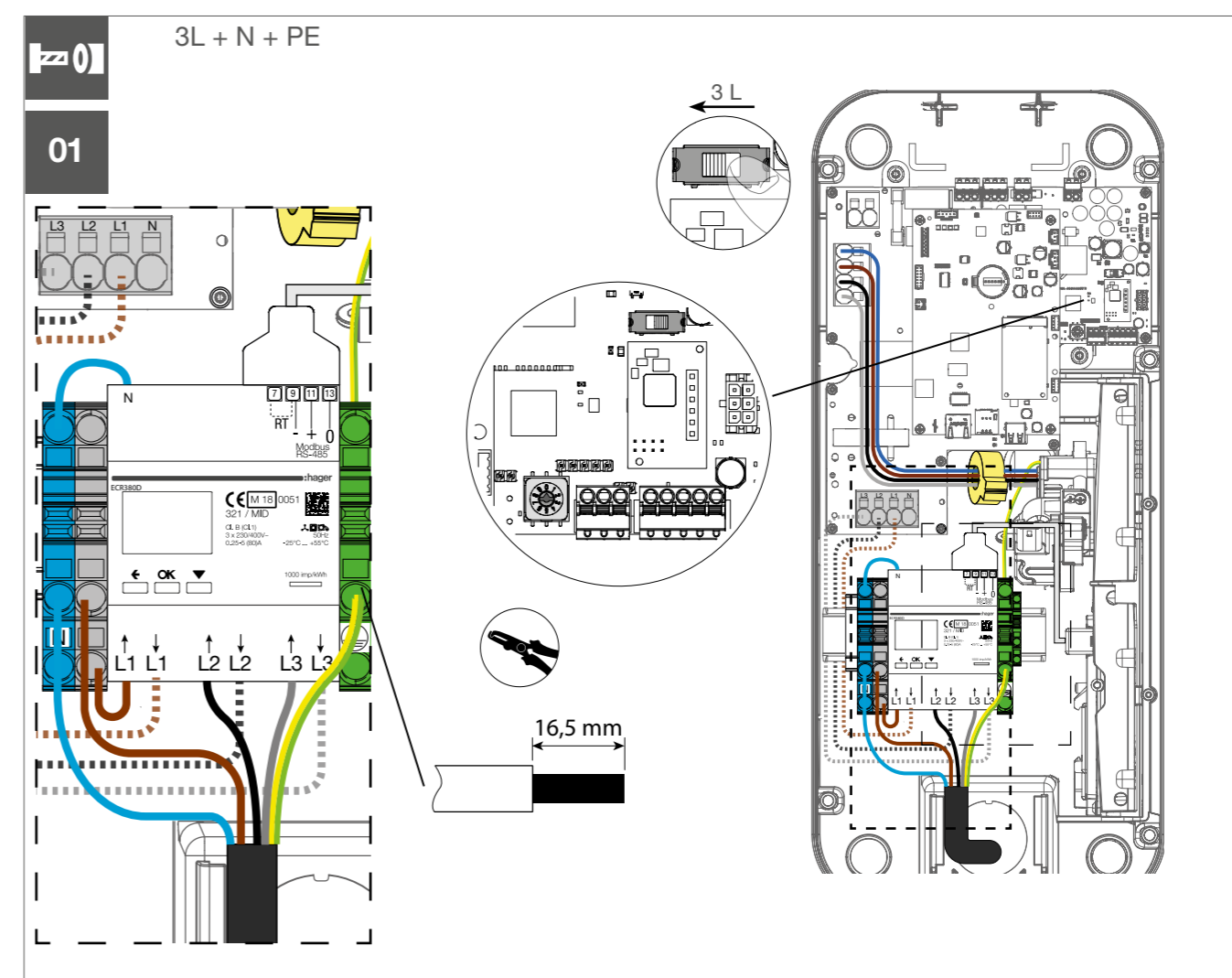
Fig 16: Elektrischer Anschluss
