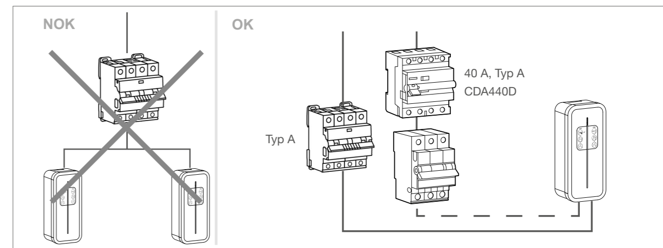
Fig 8: Anschluss 3-phasig
