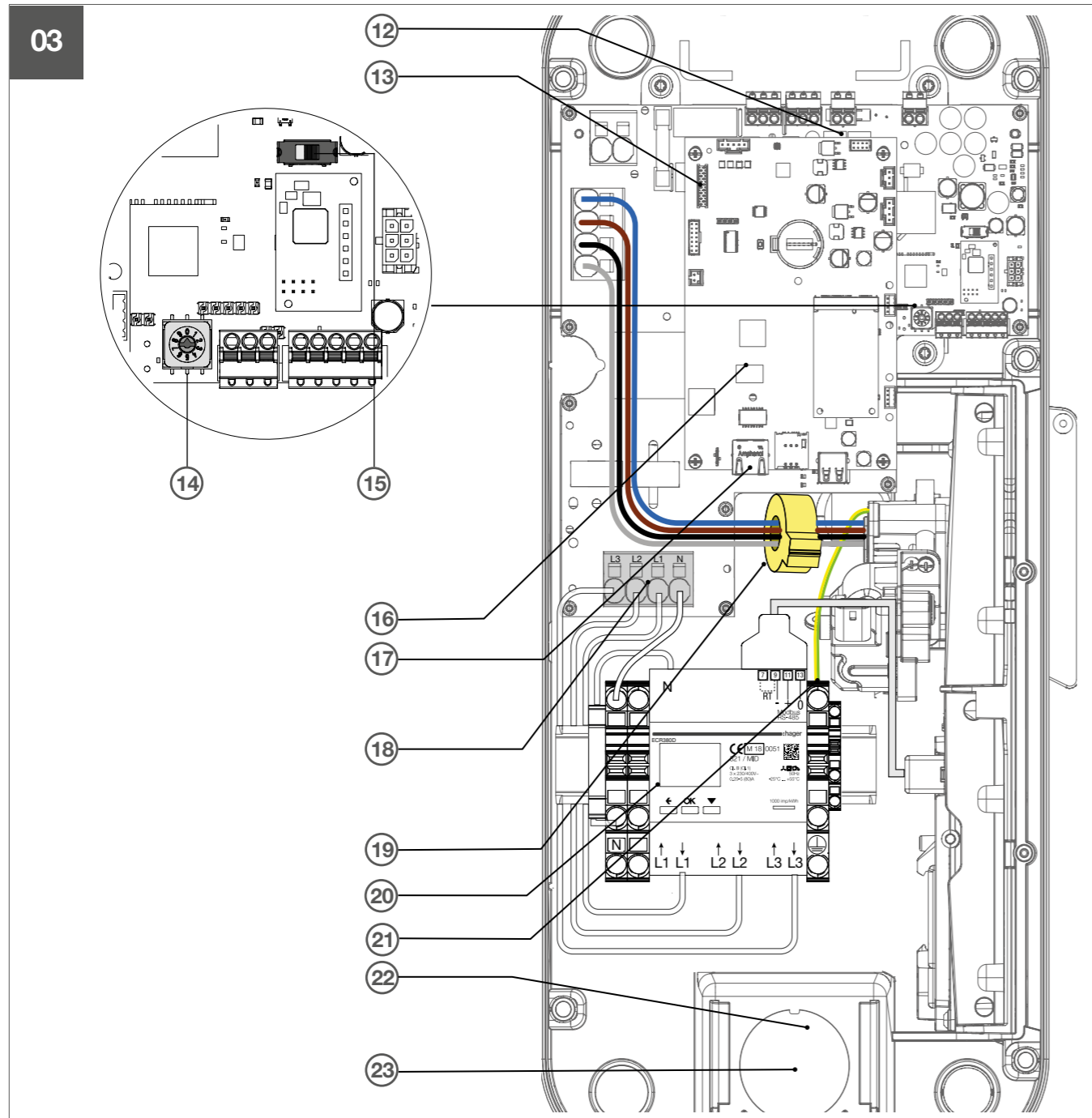
Fig 6: Elektrischer Aufbau Gerätesockel
