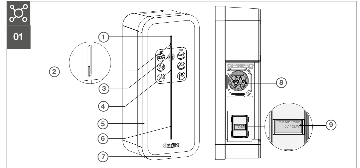
Fig 4: Geräteübersicht außen
