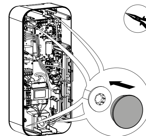
Fig 19: Endkappen montieren
