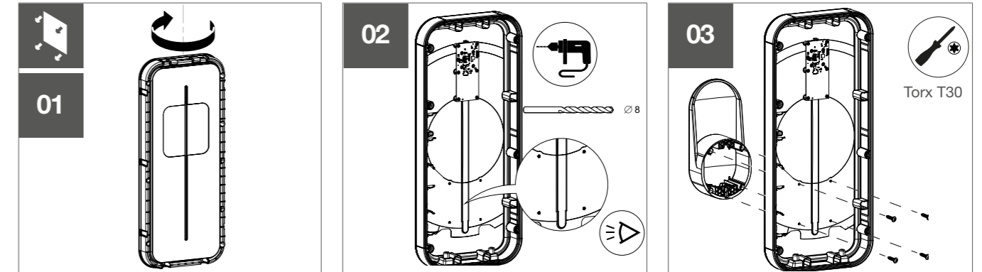
Fig 15: Montage der Kabelhalterung an der Vorderseite der Ladestation
