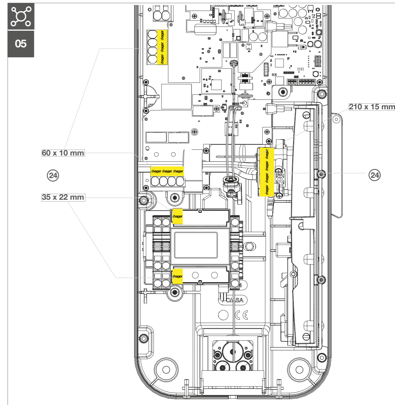
Fig 10: Sicherheitsetiketten im Geräteinneren
