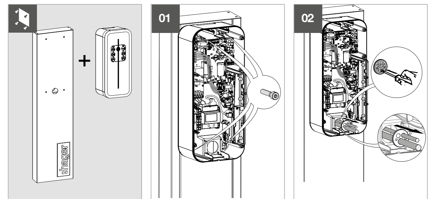
Fig 12: Standsäulenmontage
