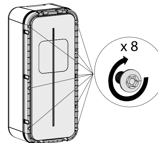
Fig 21: Gehäusedeckel verschrauben
