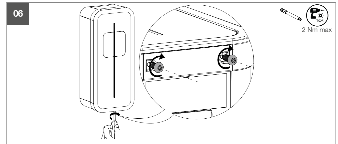
Fig 24: Montageabschluss
