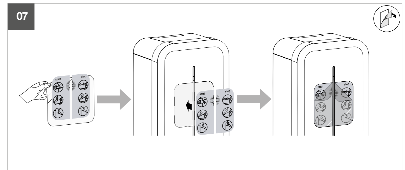
Fig 25: Bedienungsaufkleber befestigen
