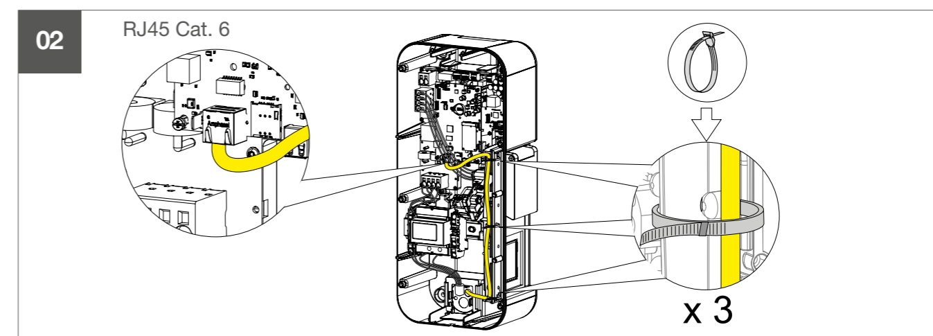
Fig 17: Anschluss Netzwerkleitung
