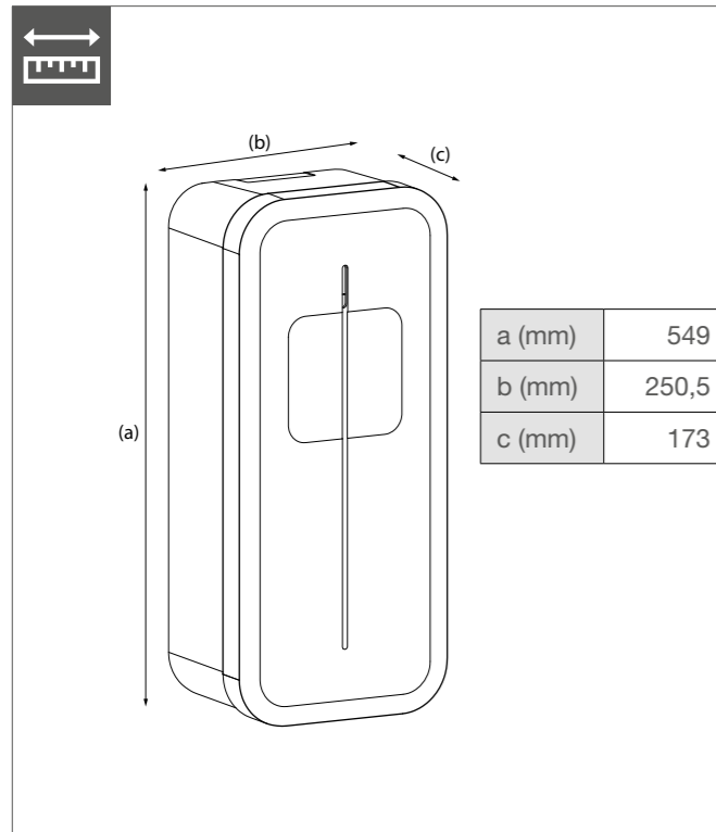
Fig 2: Abmessungen
