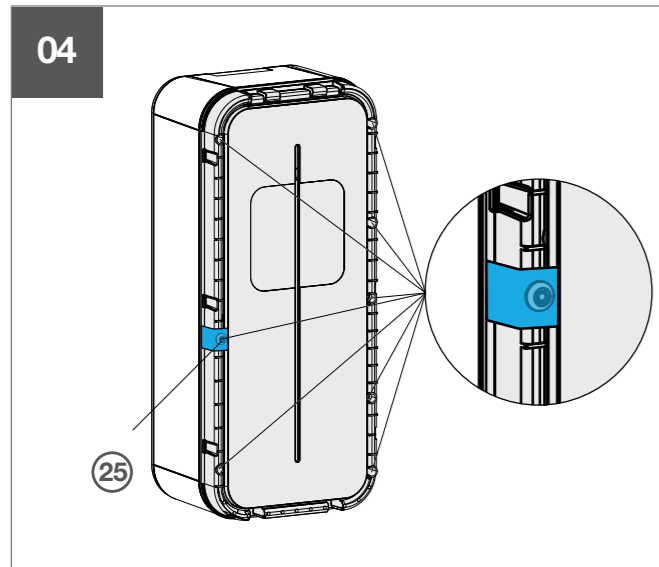
Fig 22: Sicherheitsetikett am Gehäuse anbringen
