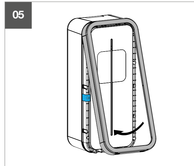
Fig 23: Kantenschutz anbringen
