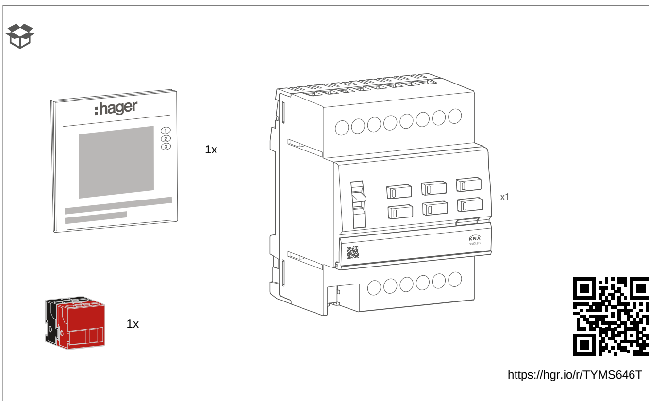
Figura 1: TYMS646T alcance de suministro
