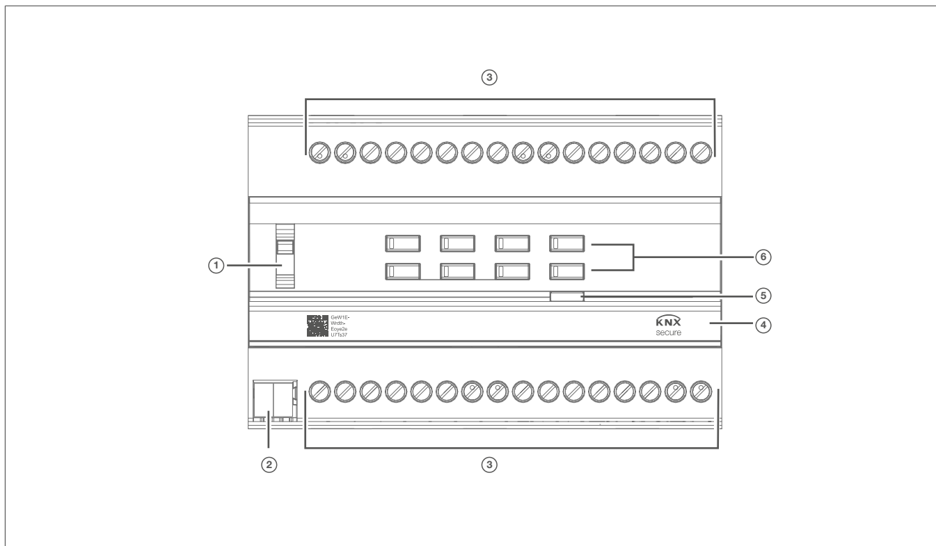
Afbeelding 2: Ontwerp en lay-out van het apparaat, schakel-/jaloezieactor, 16/8-voudig
