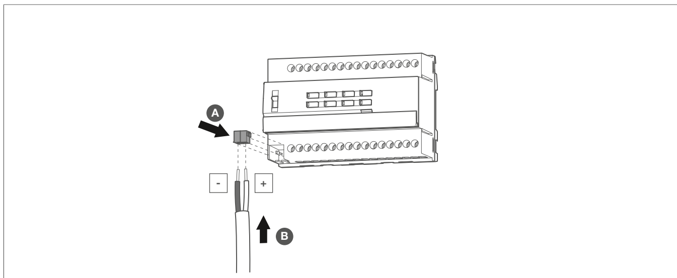
Fig. 7: Collegamento del cavo bus
