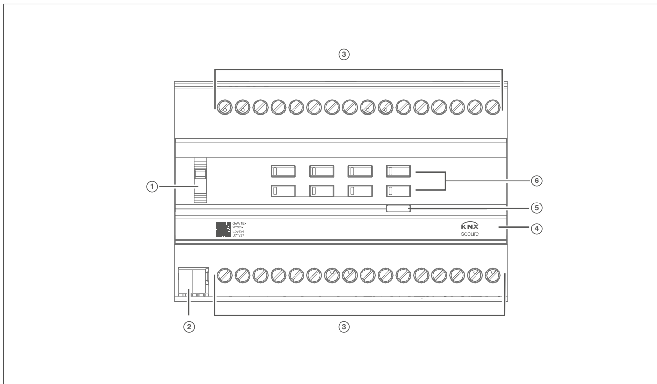
Fig. 2: Progettazione e layout del dispositivo, attuatore di commutazione ON-OFF/Veneziane-Tapparelle, 16/8 canali
