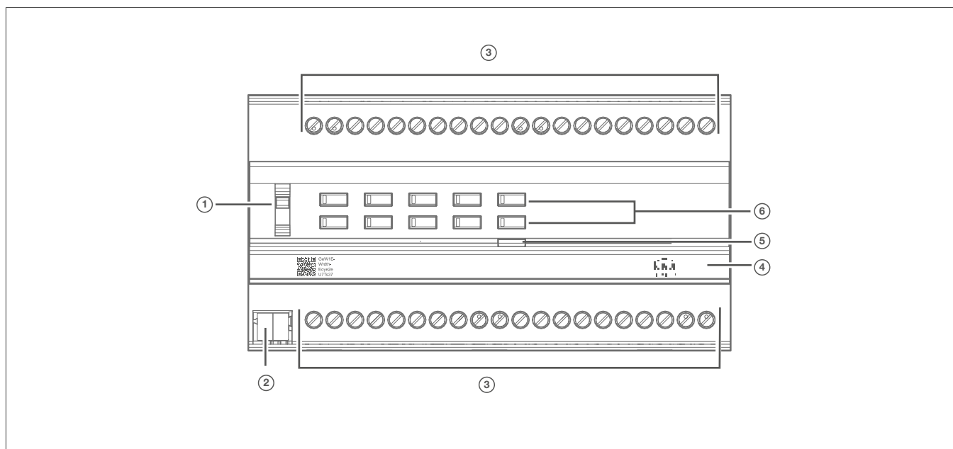
Figura 2: Diseño y estructura del dispositivo, actuador de interruptor/persiana de 20/10 elementos
