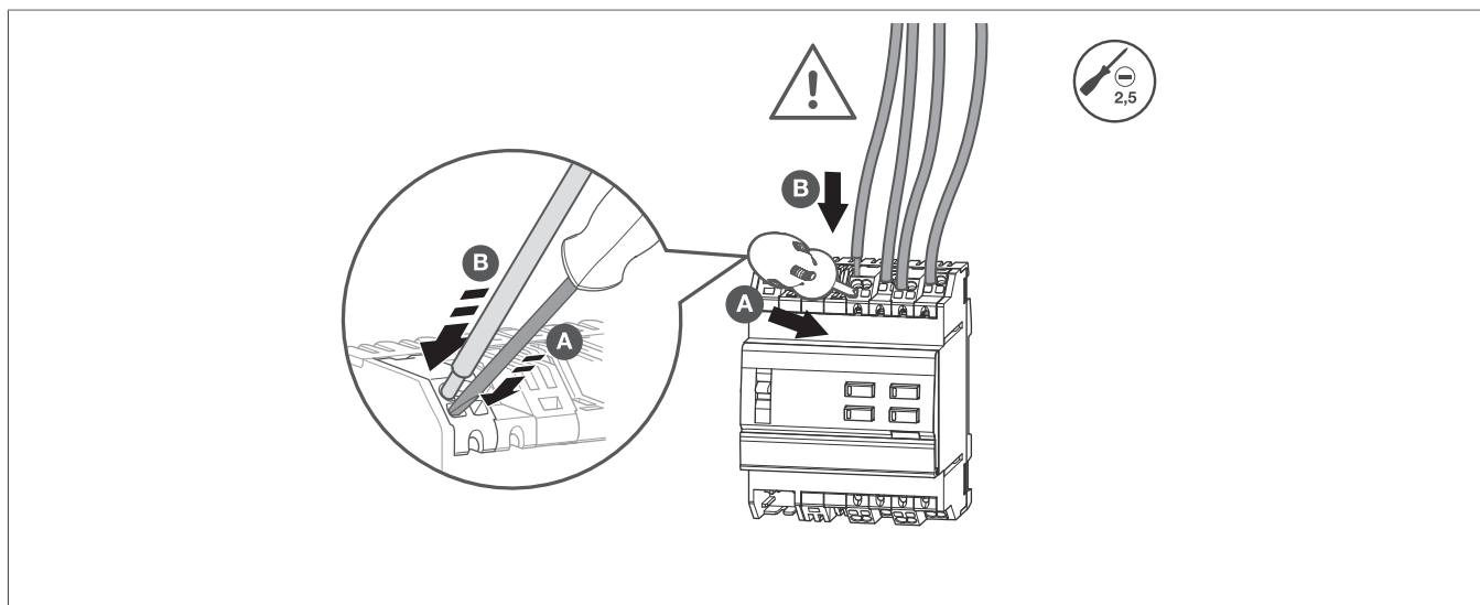
Fig. 5: Collegamento del dispositivo
