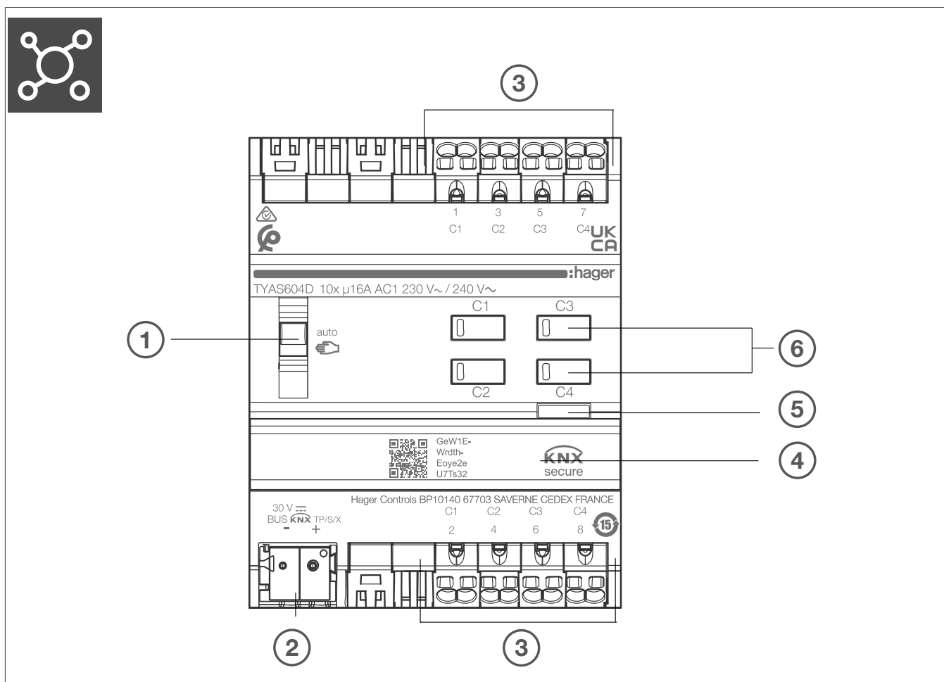
Fig. 3: Disegno e struttura del dispositivo
