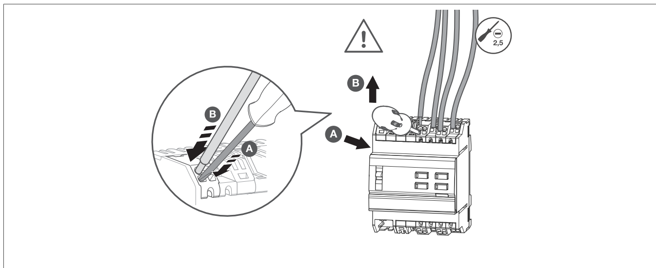
Fig. 13: Scollegamento dei cavi di collegamento
