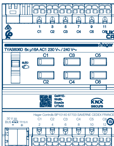
Actuador de interruptor/persiana KNX Secure de 6/3 elementos, 16 A, carga C TYAS606D
