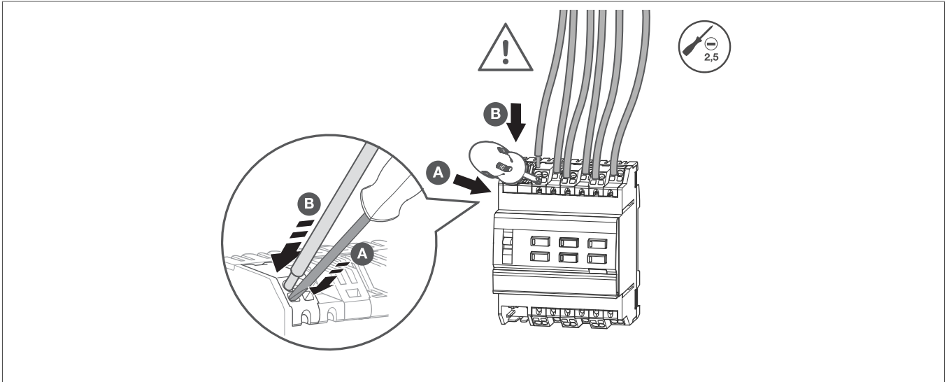
Figura 5: Conexión del dispositivo
