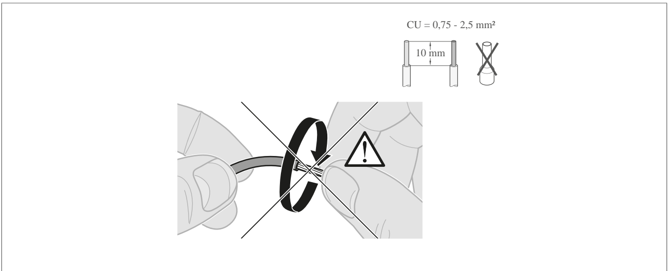
Figura 6: Longitud de pelado y sección de cable
