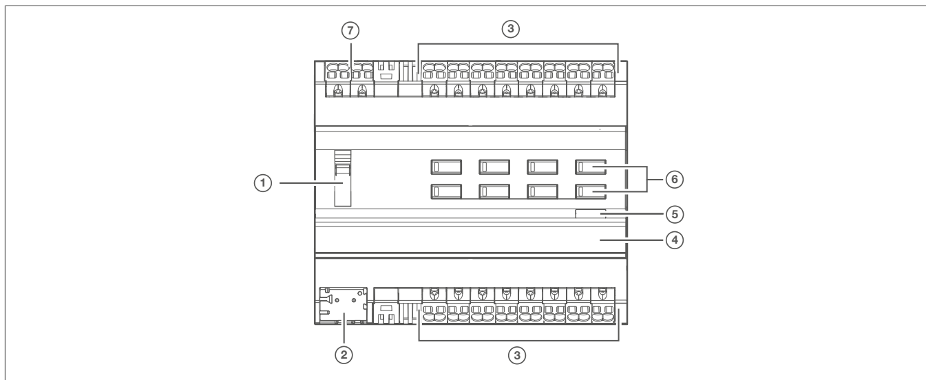
Figura 3: Diseño y estructura del dispositivo
