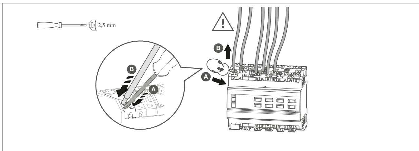
Figura 13: Desconectar los cables de conexión
