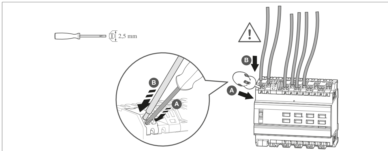
Figura 5: Conexión del dispositivo
