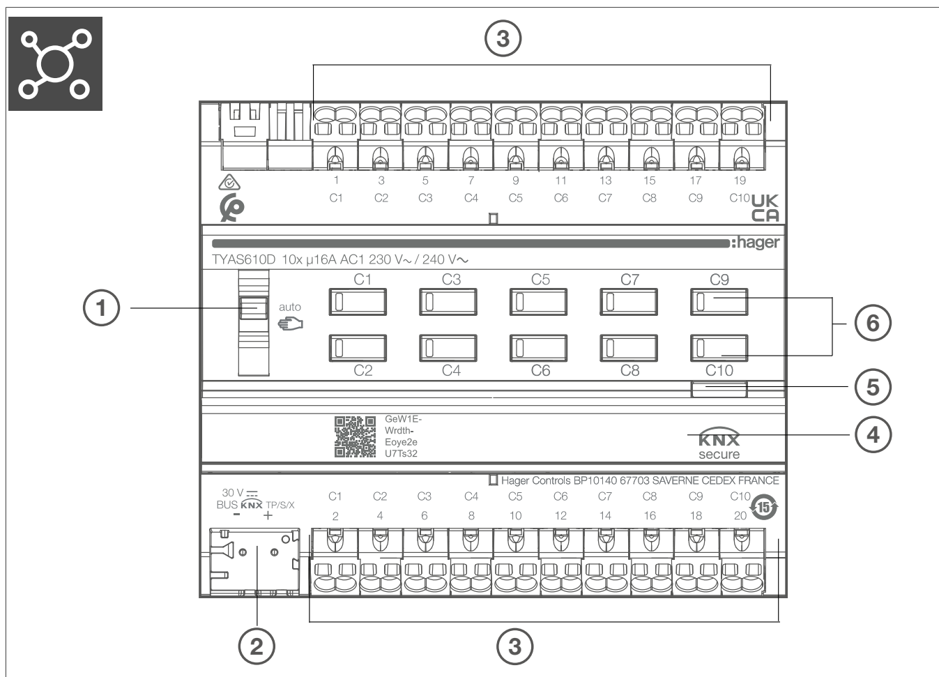
Figura 2: Diseño y estructura del dispositivo
