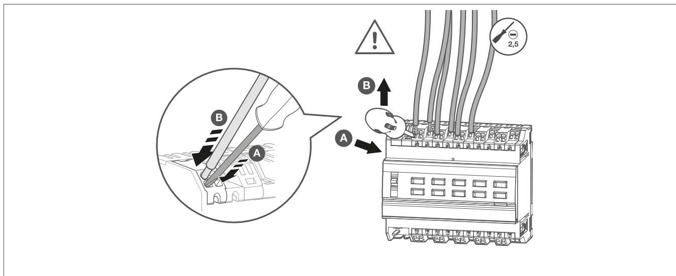
Figura 12: Desconectar los cables de conexión
