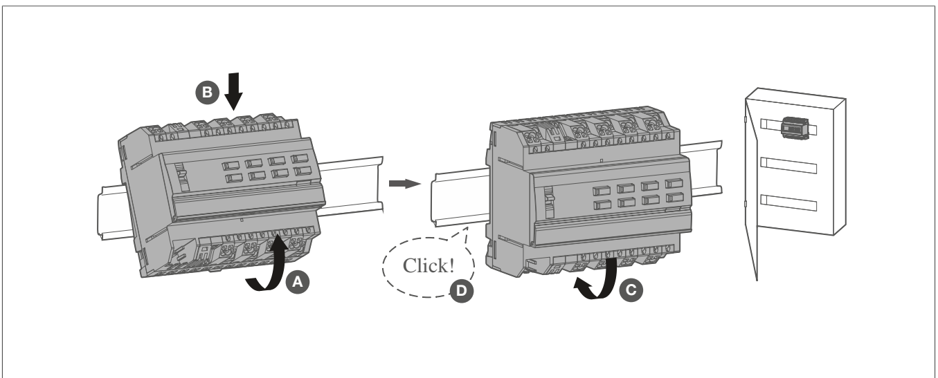
Figura 3: Instalación del dispositivo en el carril DIN
