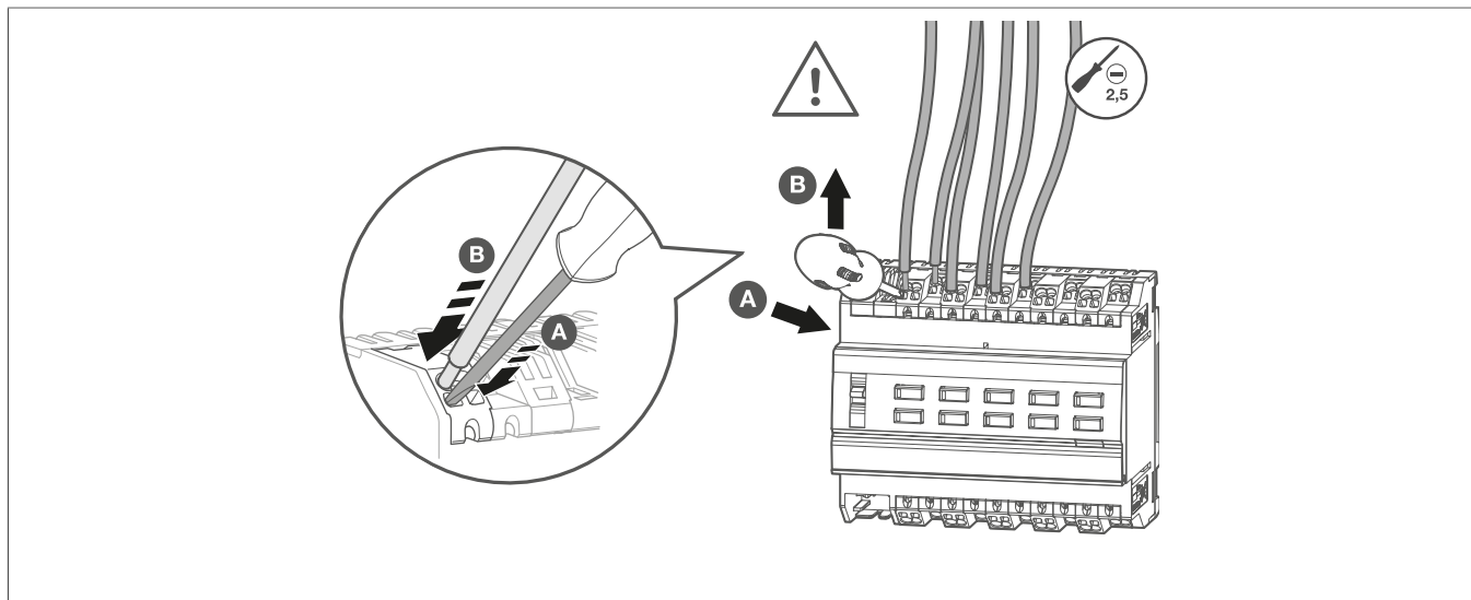
Figura 4: Conexión del dispositivo
