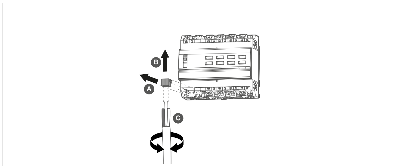
Figura 13: Remover o terminal de ligação de bus
