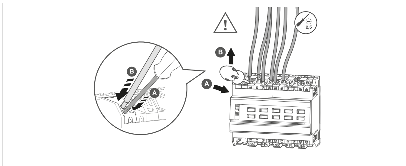
Figura 12: Desligar os cabos de ligação
