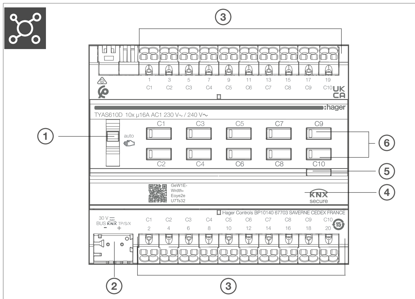
Figura 2: Desenho e esquema de ligações do aparelho
