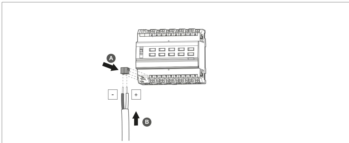
Figura 6: Ligar o terminal de ligação de bus
