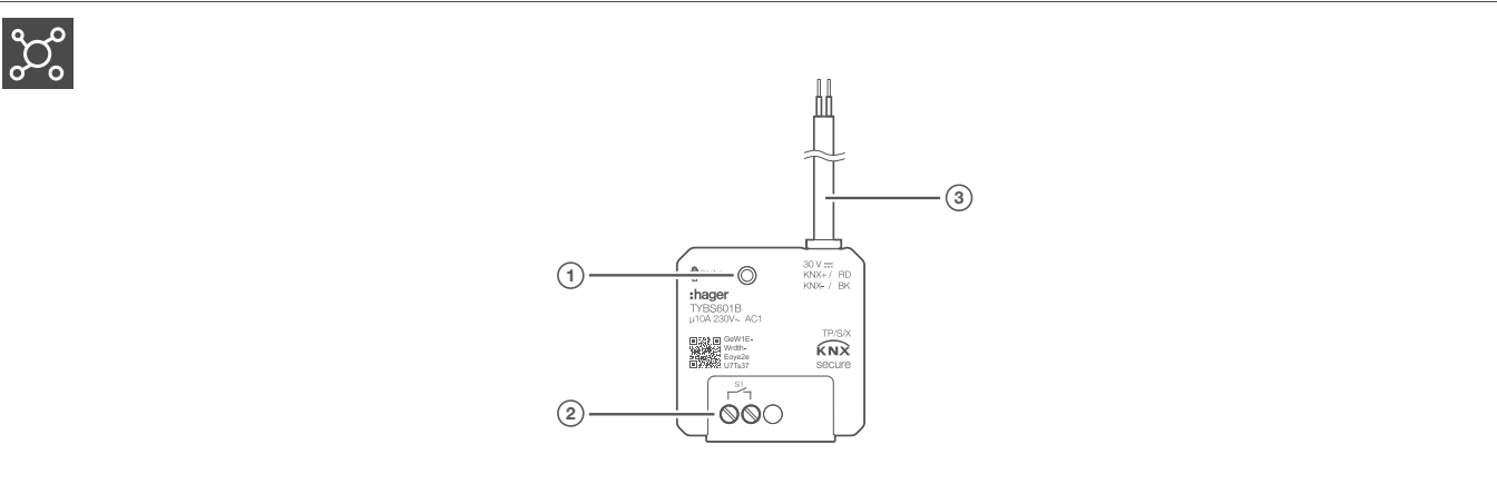
Figura 2: Diseño y estructura del dispositivo TYBS601B
