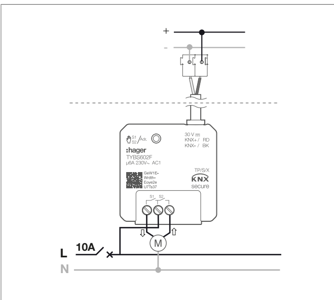
Fig. 4 : Schéma de raccordement de la charge moteur TYBS602Fli
