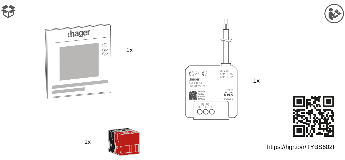
Fig. 1 : Contenu de la livraison TYBS602F
