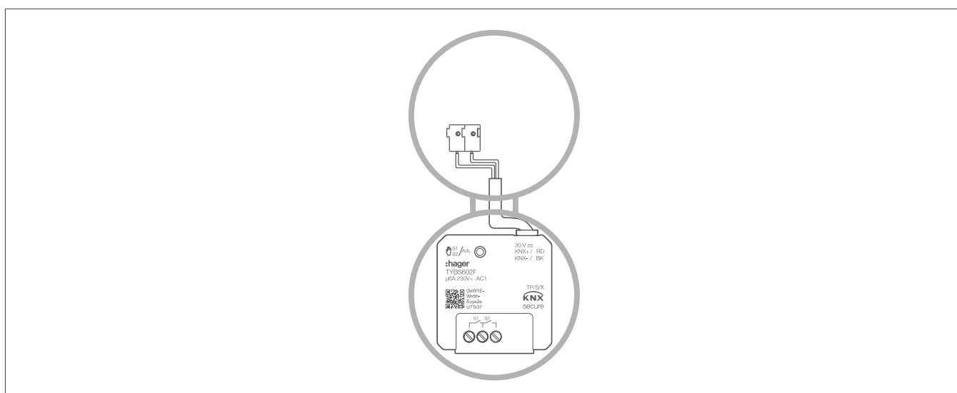
Fig. 5 : Montage dans un boîtier d'encastrement mural double
