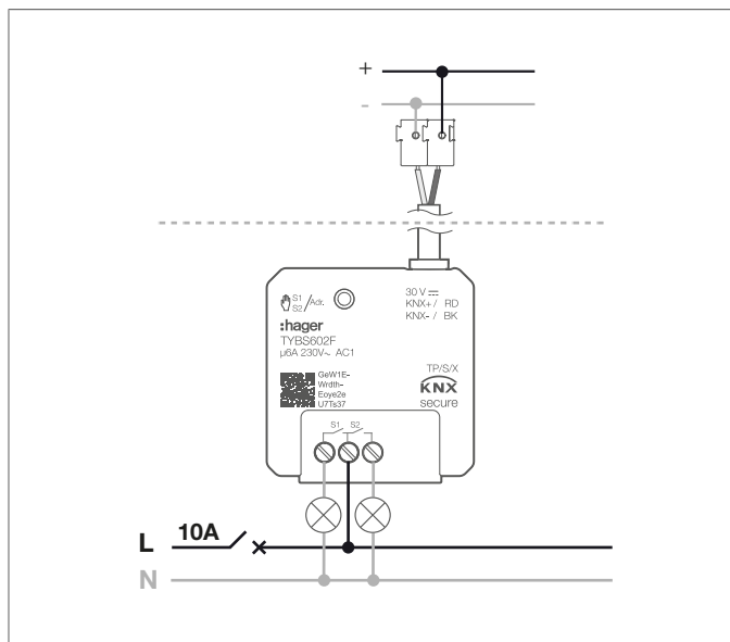
Figura 3: TYBS602F diagrama de conexión de carga de lámpara
