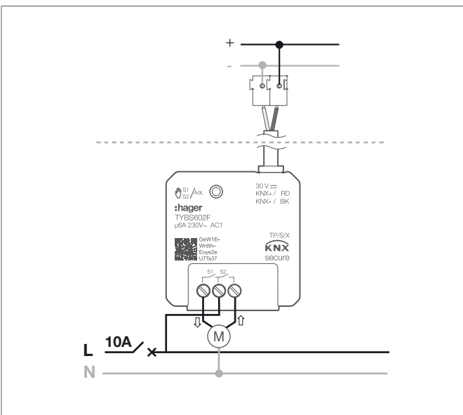
Figura 4: TYBS602F diagrama de conexión de carga del motor
