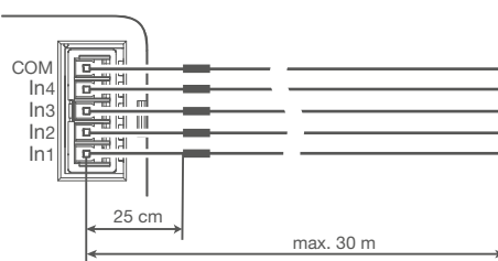
Bild 4: Max. Leitungslänge pro Leitungssatz
