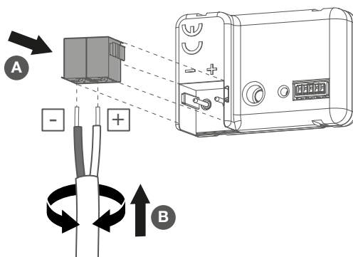
Bild 3: Busleitung anschließen
