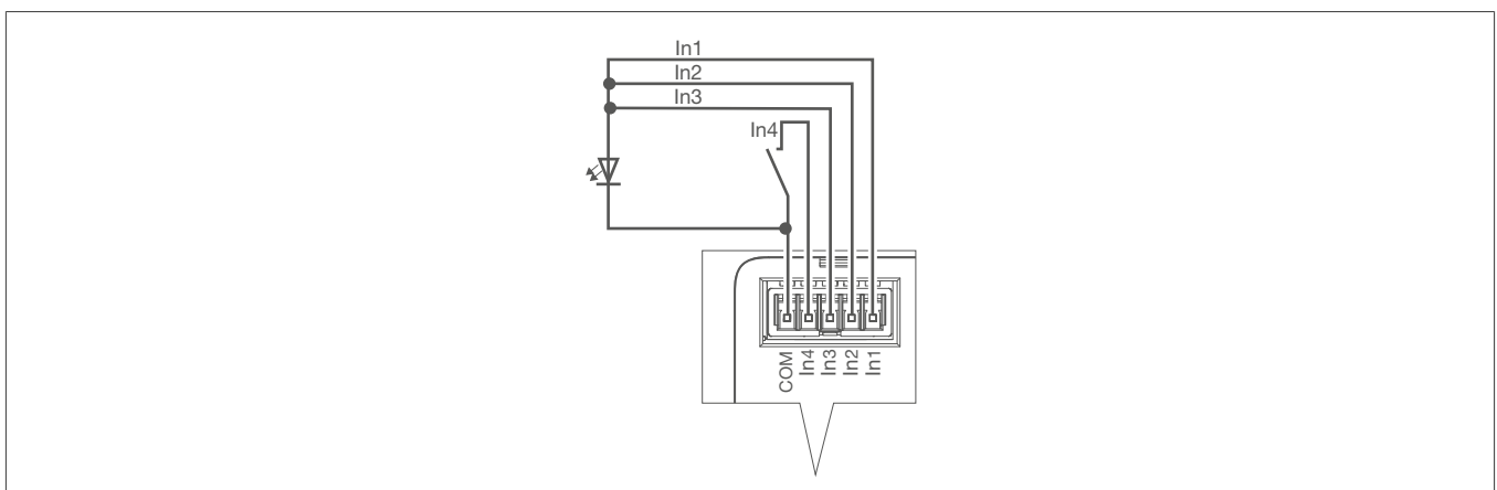
Bild 6: Anschlussbeispiel parallelgeschalteter Ausgänge
