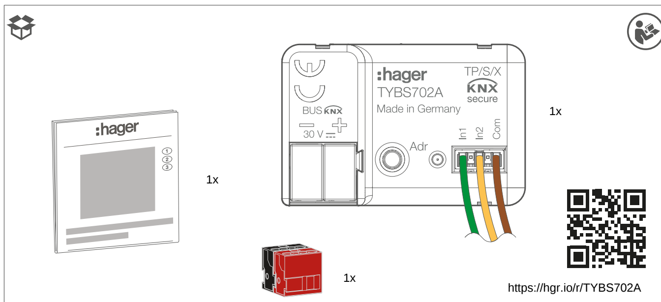
Bild 1: Lieferumfang TYBS702A
