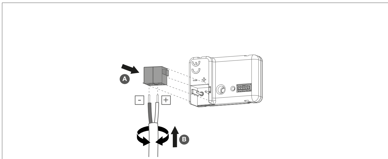
Fig. 2 : Raccordement du câble de bus
