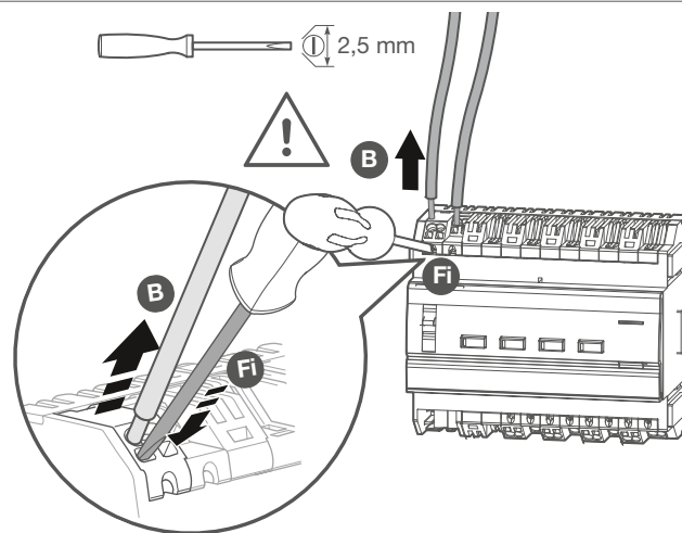
Fig. 9: Scollegamento dei cavi di collegamento
