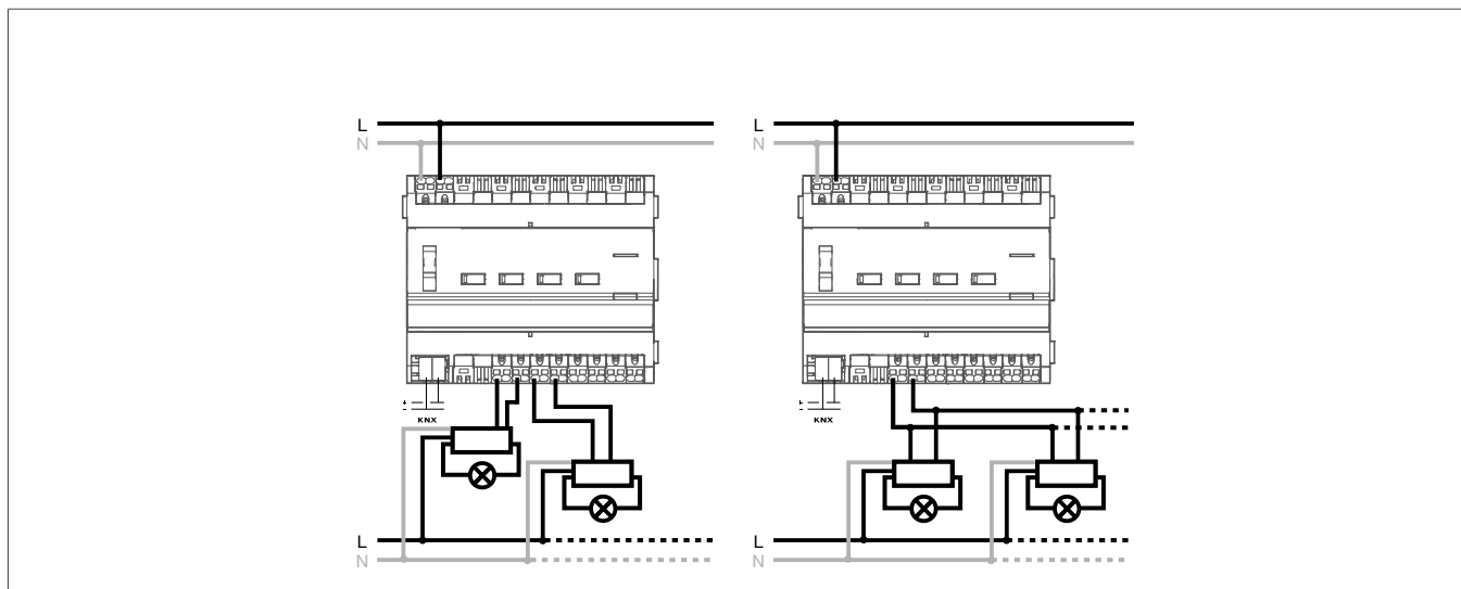
Fig. 7: Collegamento del carico al dispositivo
