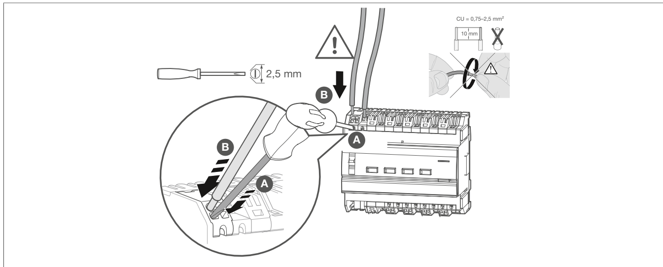
Fig. 6: Collegamento del dispositivo
