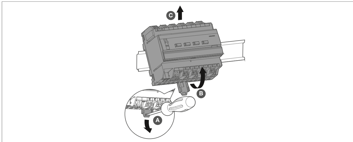
Fig. 11: Rimozione del dispositivo dalla guida DIN
