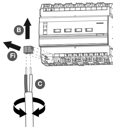
Fig. 10: Rimozione del morsetto di collegamento bus
