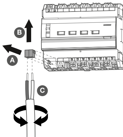
Afbeelding 10: De busverbindingsklemmen verwijderen
