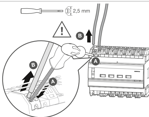
Afbeelding 9: Loskoppelen van de verbindingkabels
