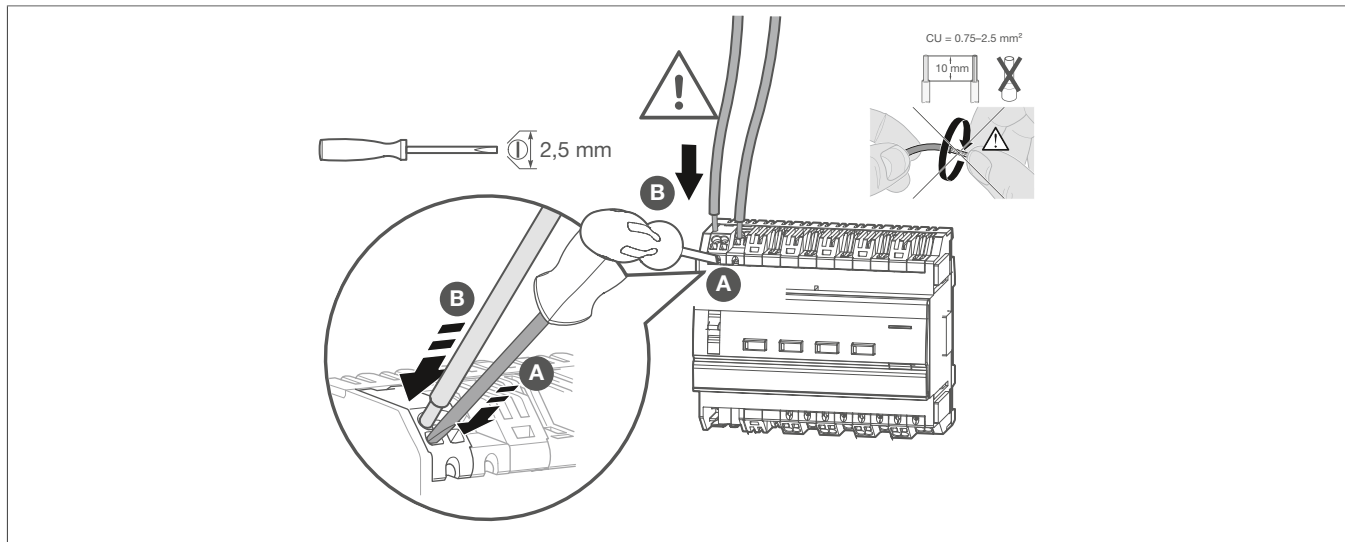
Figura 6: Conexión del dispositivo
