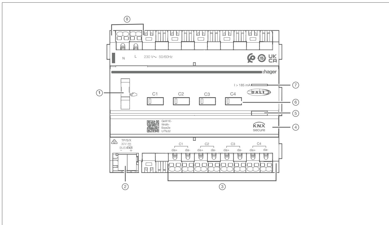
Figura 2: Diseño y estructura del dispositivo TYAS664D
