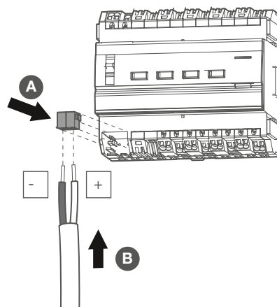
Figura 8: Conectar el cable bus
