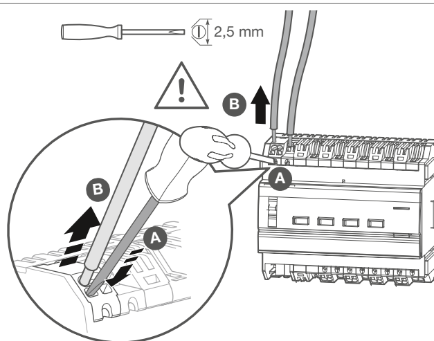
Figura 9: Desconectar los cables de conexión
