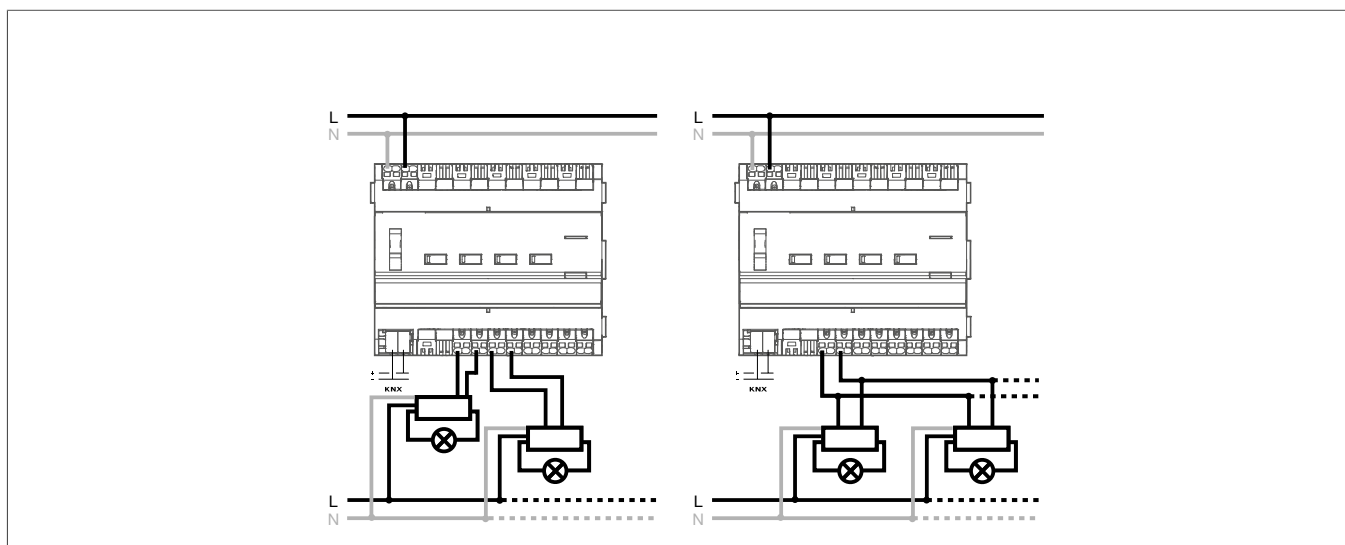
Figura 7: Conectar la carga al dispositivo
