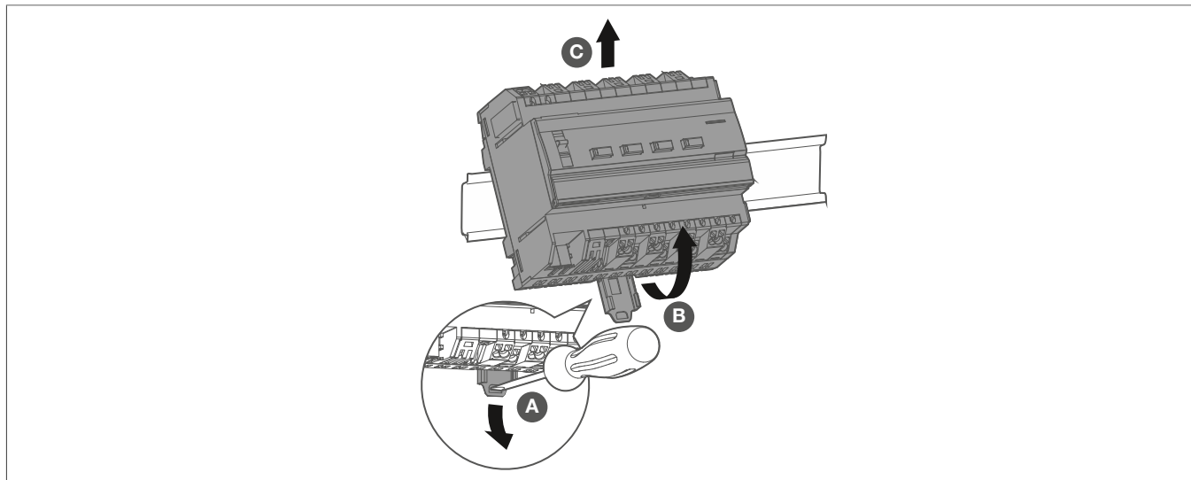
Figura 11: Fijar el dispositivo en el carril DIN.
