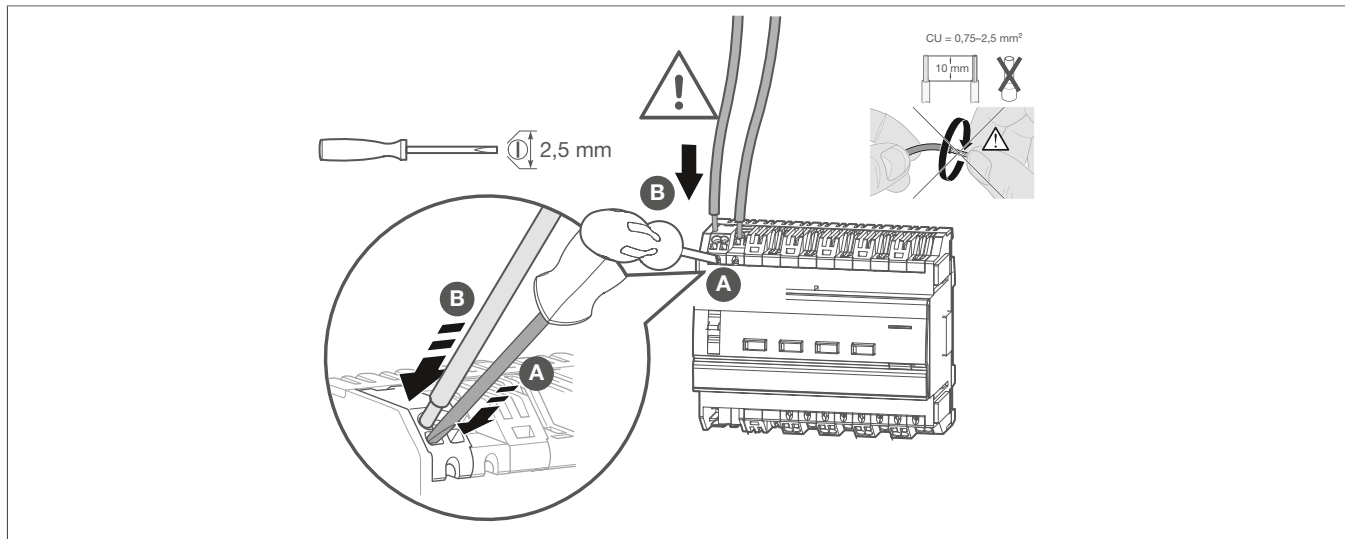
Figura 6: Ligar o produto
