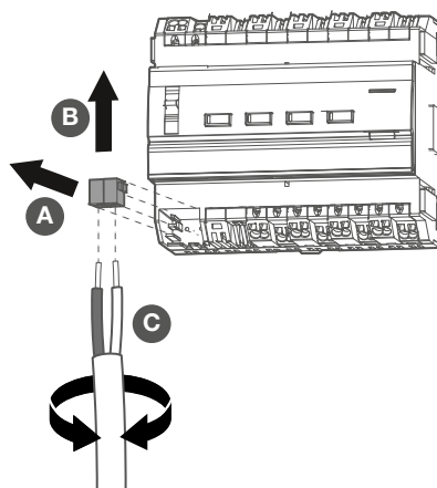
Figura 10: Remover o terminal de ligação de bus
