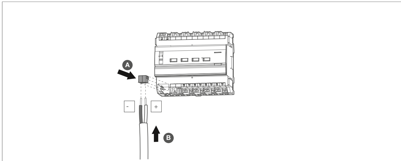
Figura 8: Ligação do cabo de bus
