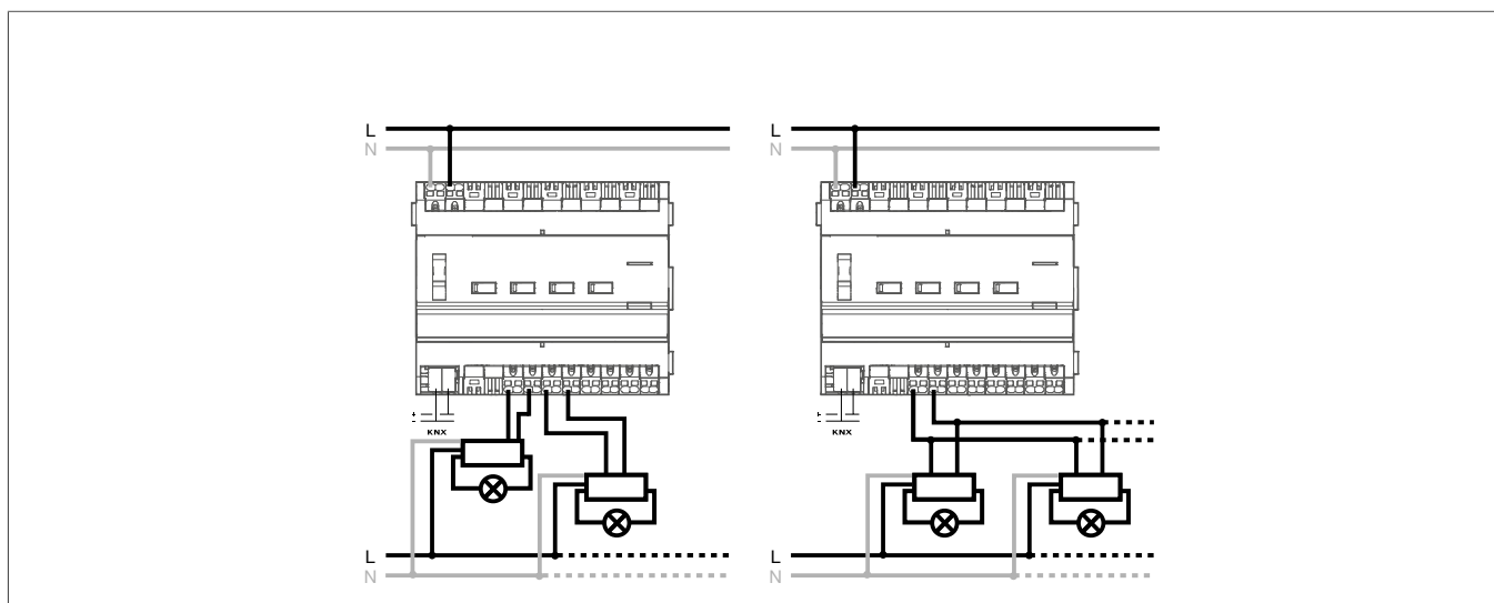
Figura 7: Ligação da carga ao produto
