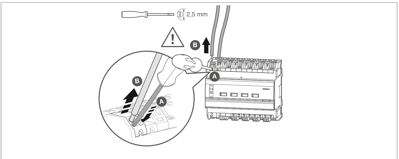
Bild 10: Anschlussleitungen abklemmen
