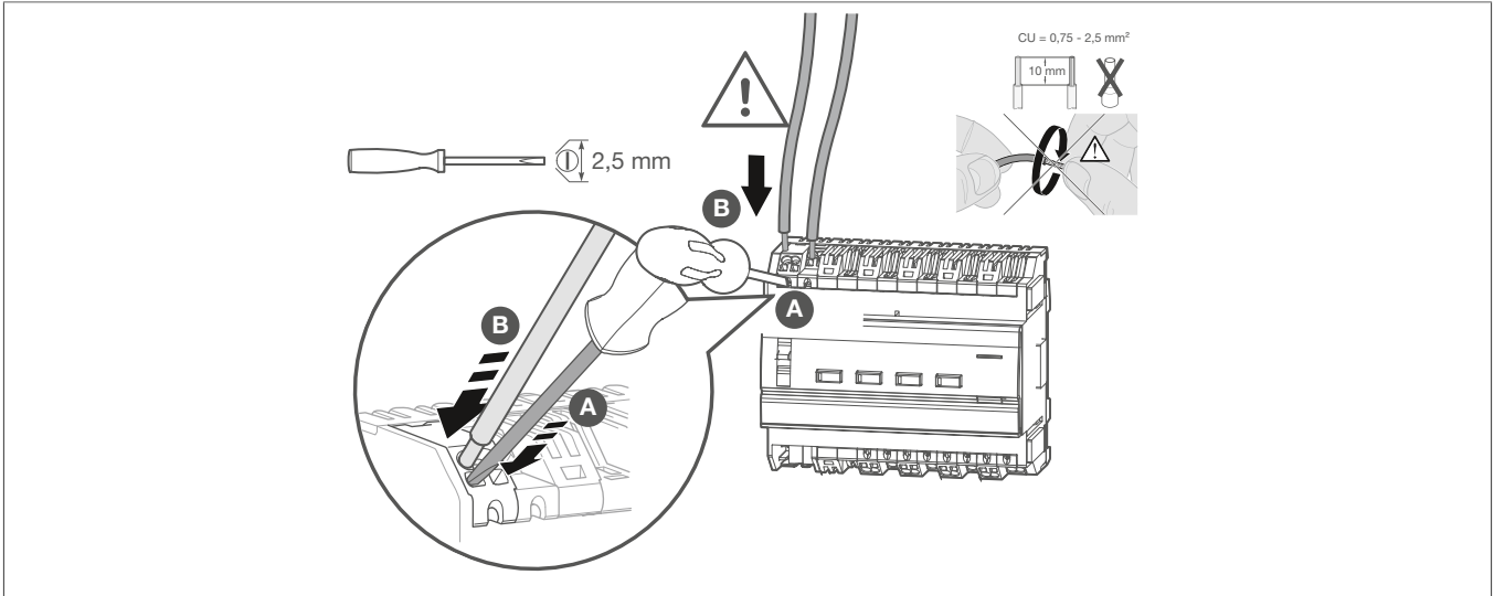
Bild 6: Gerät anschließen
