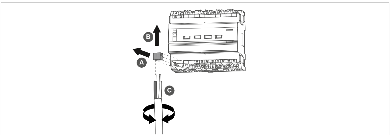
Bild 11: Busanschlussklemme abziehen
