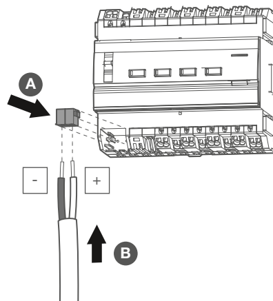
Bild 8: Busleitung anschließen
