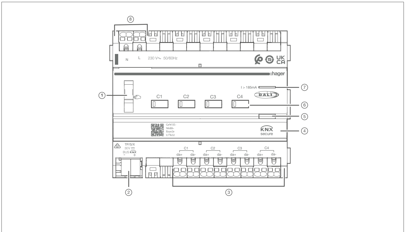
Bild 2: Geräteaufbau TYAS664D
