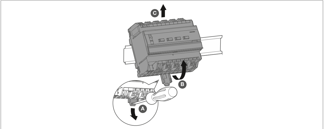
Bild 12: Gerät von der Hutschiene montieren
