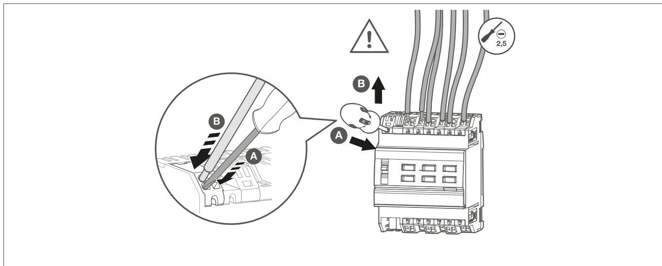
Fig. 10: Scollegamento dei cavi di collegamento
