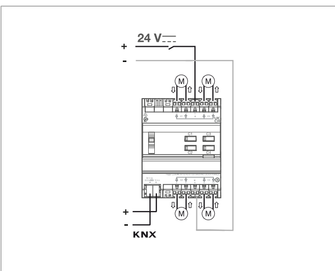
Fig. 3: Collegamento del dispositivo
