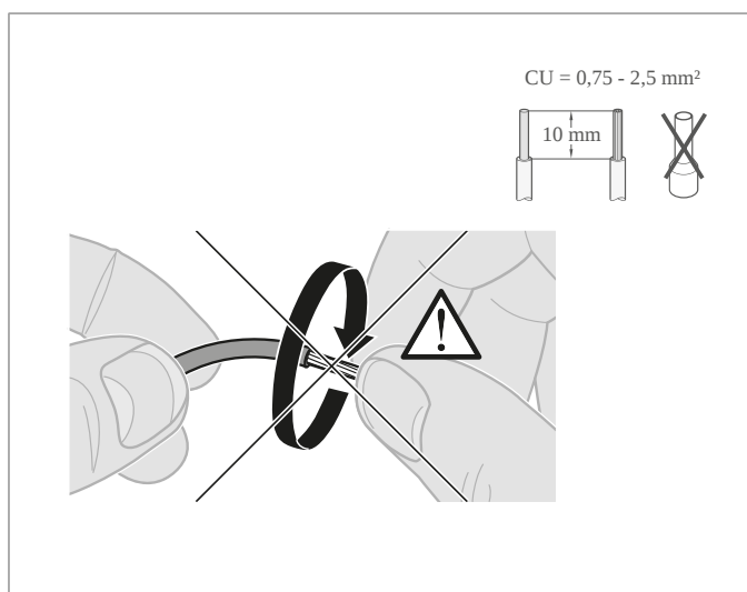
Fig. 2: Preparare le linee di allacciamento.
