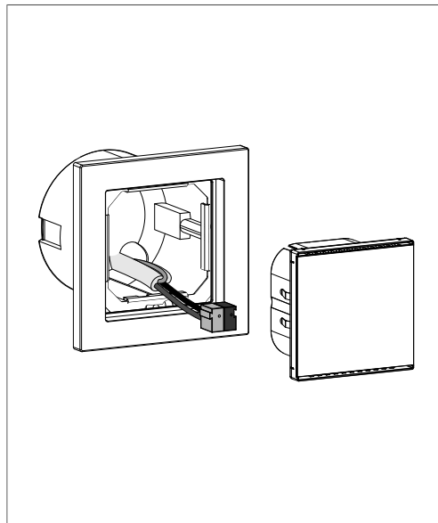
Bild 4: Rahmen und Modul montieren
