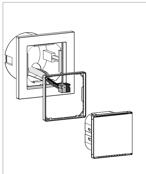
Bild 6: Rahmen, Adapterring und Modul montieren
