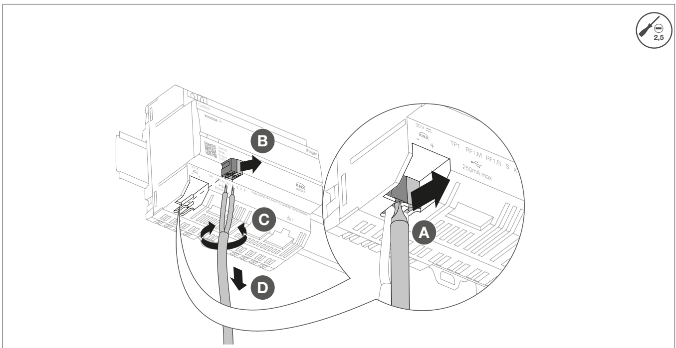
Bild 15: Busanschlussklemme abziehen
