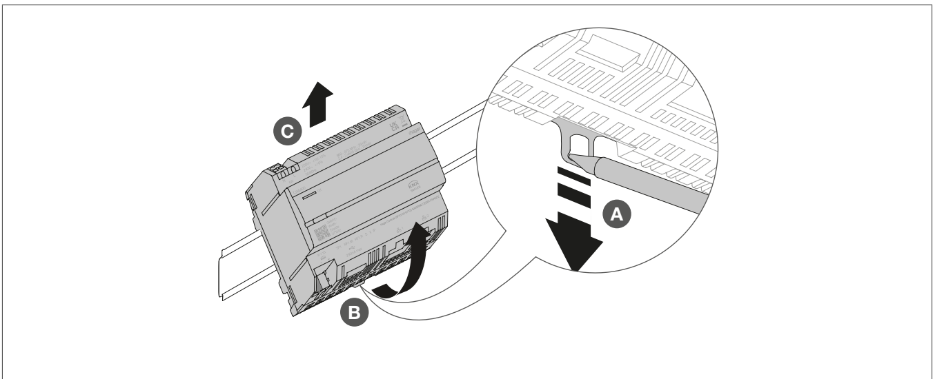
Bild 17: Gerät von der Hutschiene montieren
