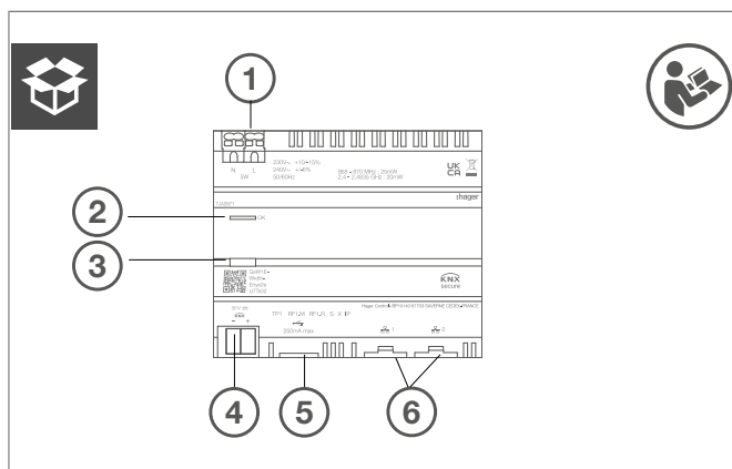
Bild 5: Geräteaufbau - Draufsicht
