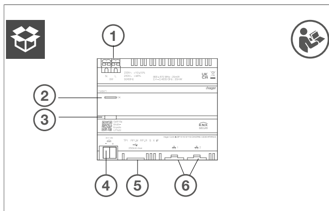
Bild 3: Geräteaufbau - Draufsicht
