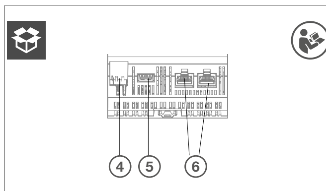
Bild 6: Geräteaufbau - Ansicht von unten auf KNX-, USB- und Ethernet-Schnittstellen
