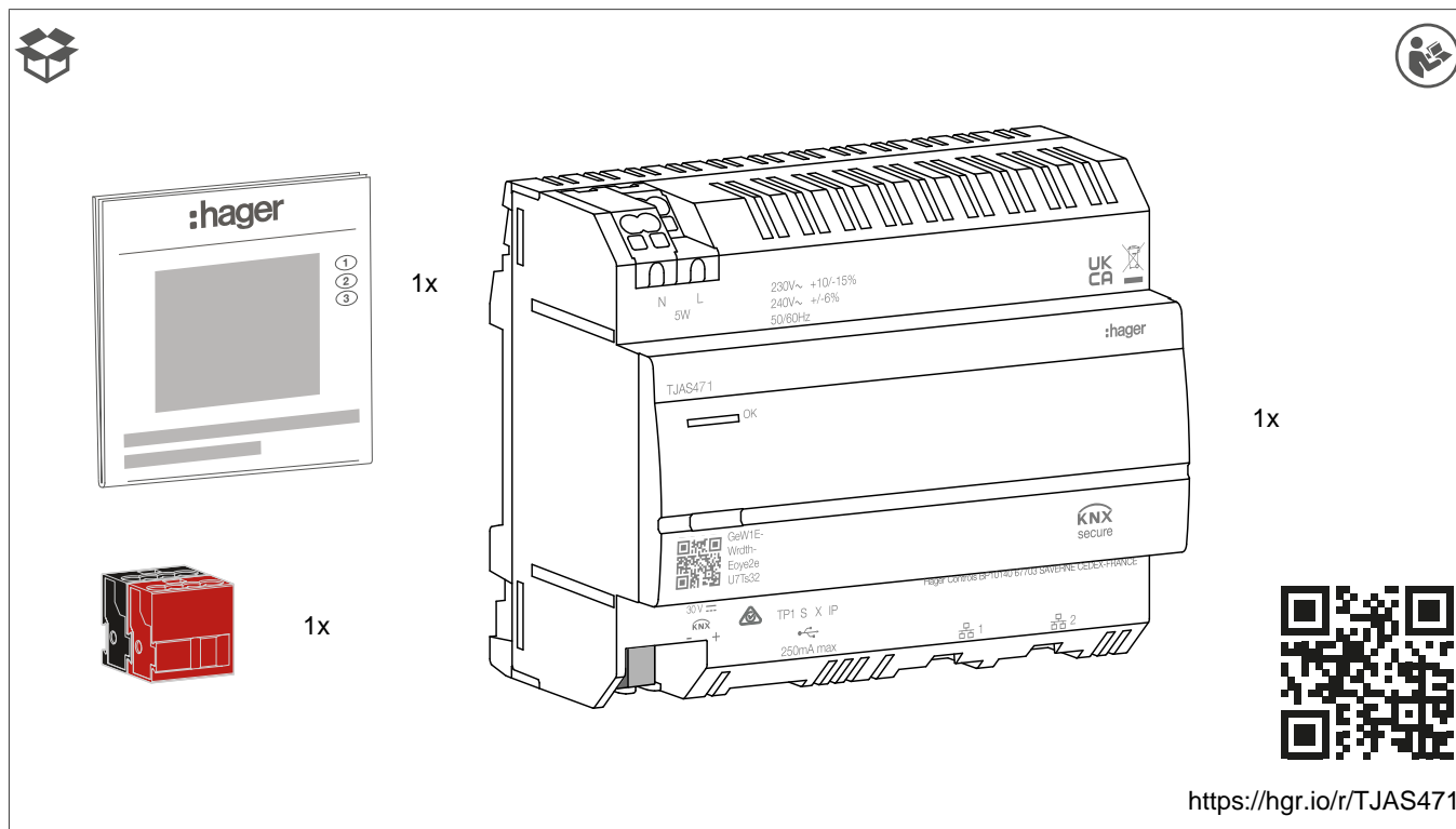
Bild 1: Lieferumfang TJAS471
