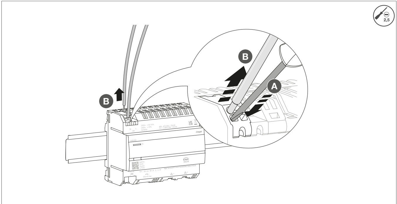
Bild 14: Anschlussleitungen abklemmen
