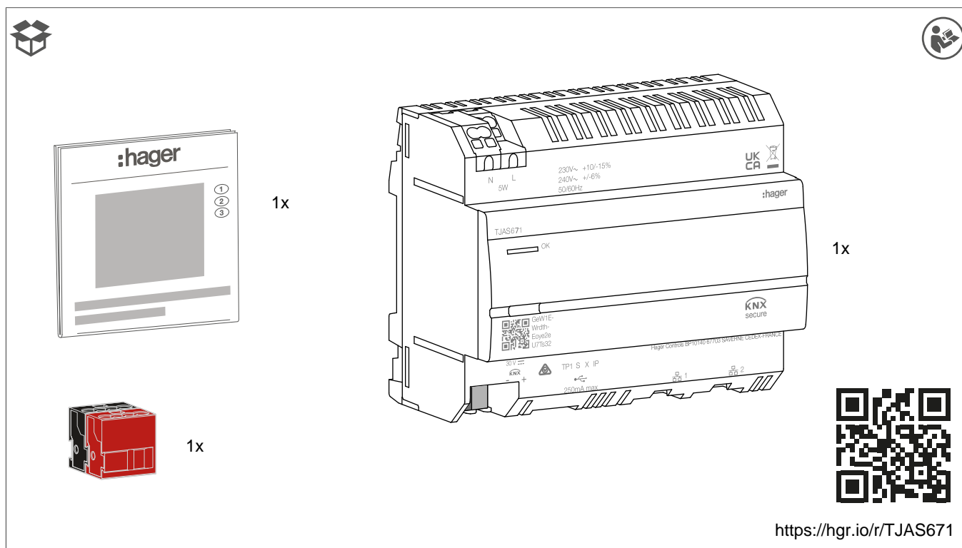
Bild 2: Lieferumfang TJAS671
