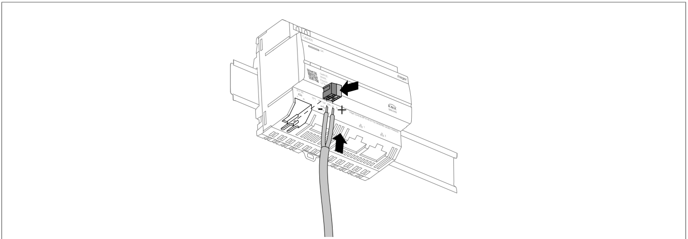
Bild 13: Busleitung anschließen
