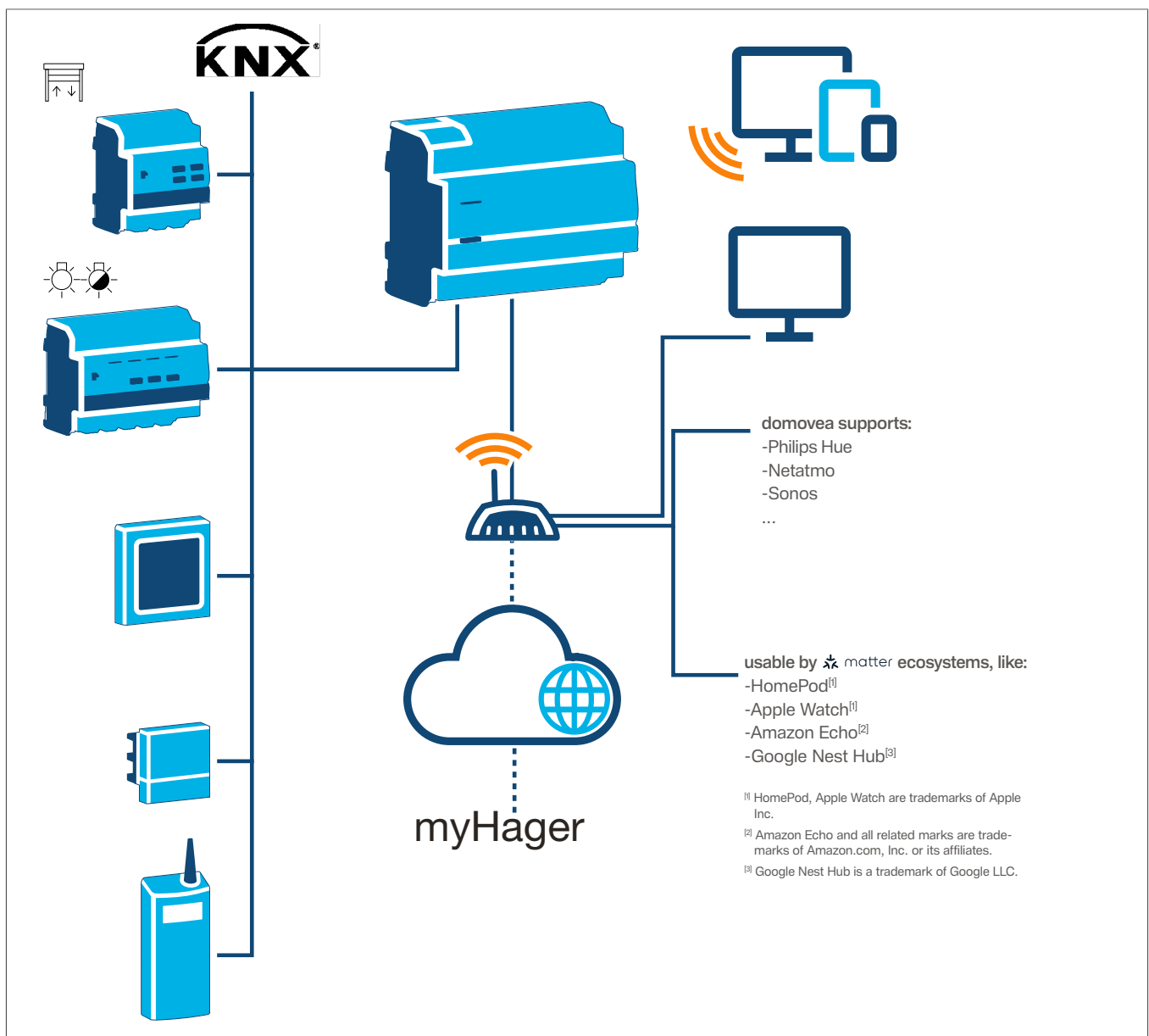
Bild 7: Systemübersicht
