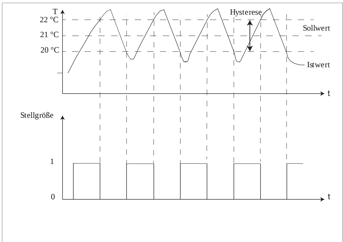
Bild 18: 2Punkt-Regelung
